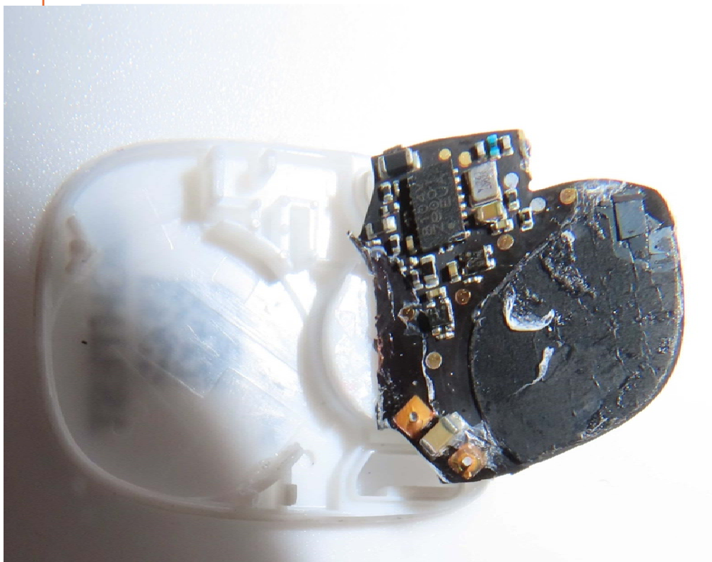
NFC Antenna
