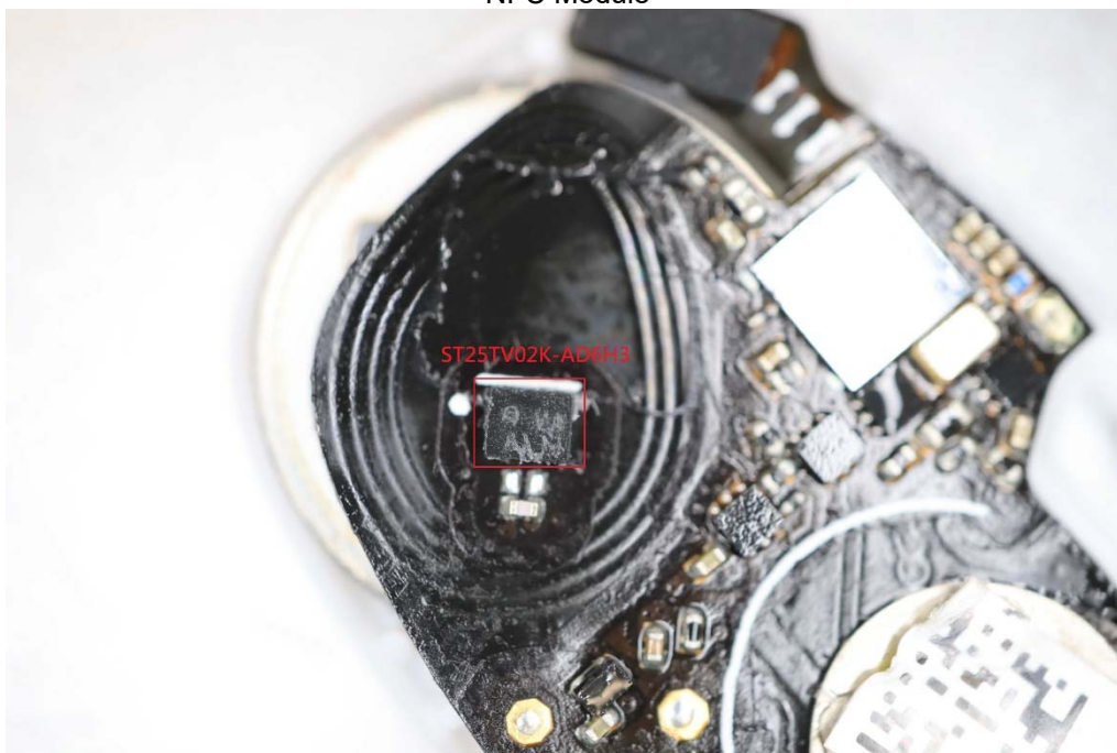
NFC Module
