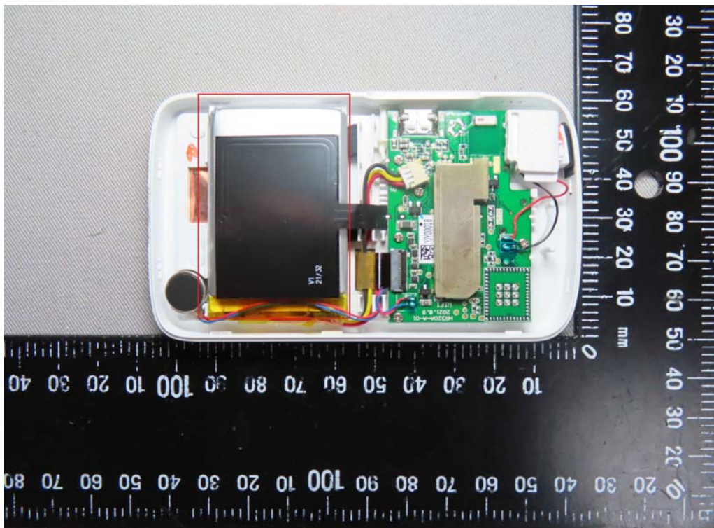
NFC Antenna
