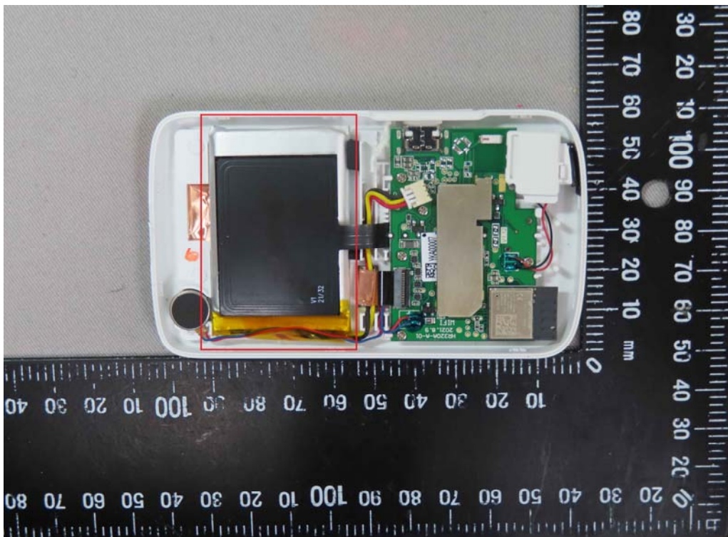
NFC Antenna
