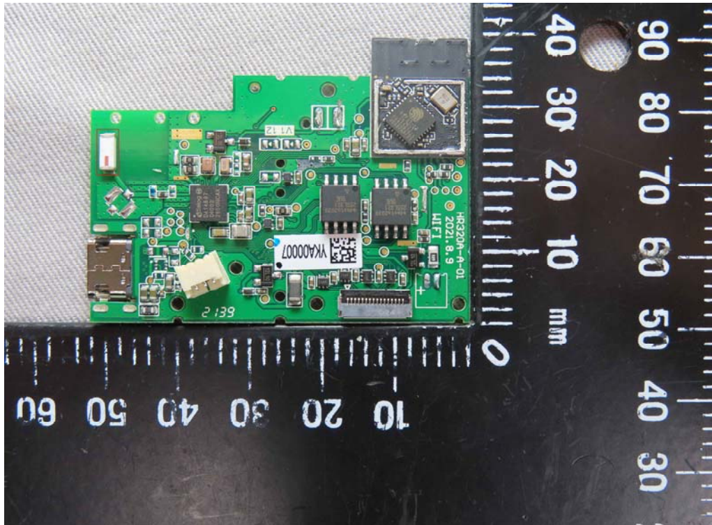
BLE Antenna
