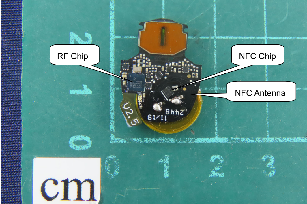
(74) EUT Photo
