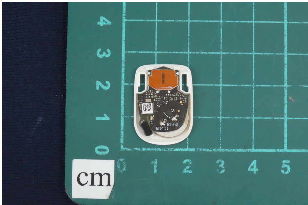
(57) EUT Photo
