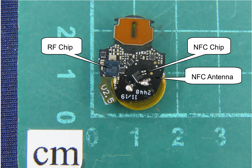
(70) EUT Photo
