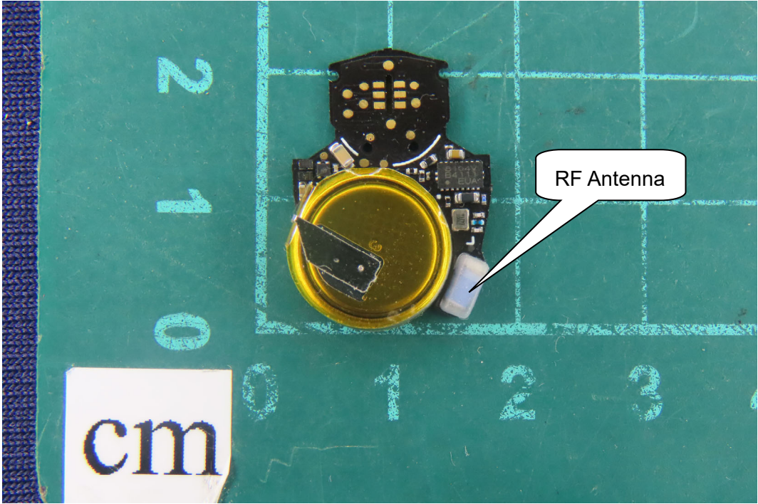
(75) EUT Photo
