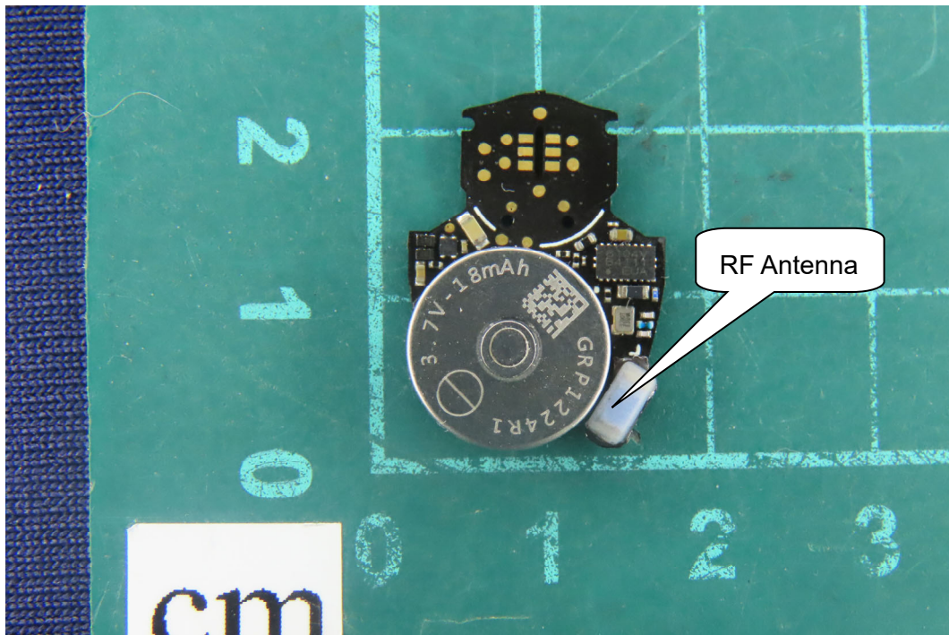
(63) EUT Photo
