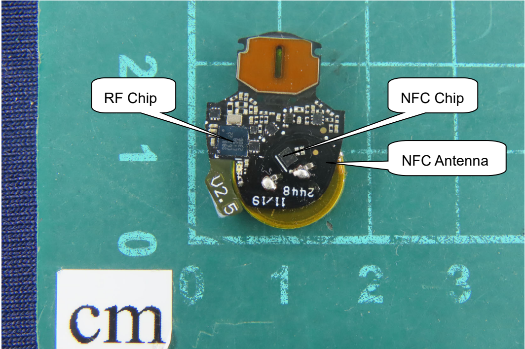
(78) EUT Photo
