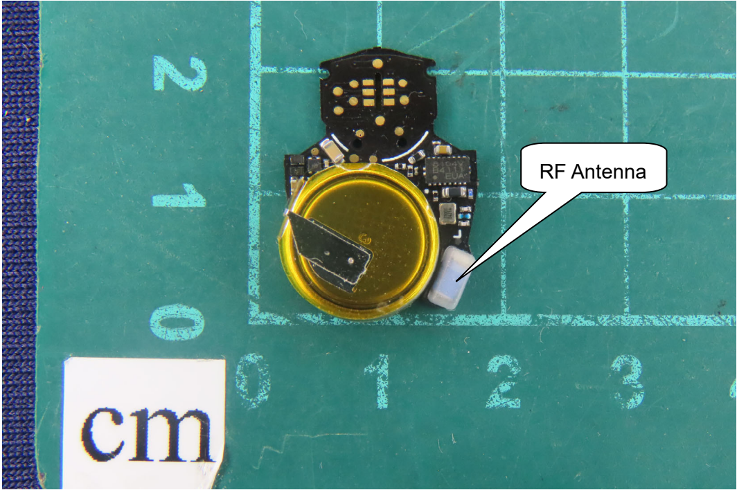
(83) EUT Photo
