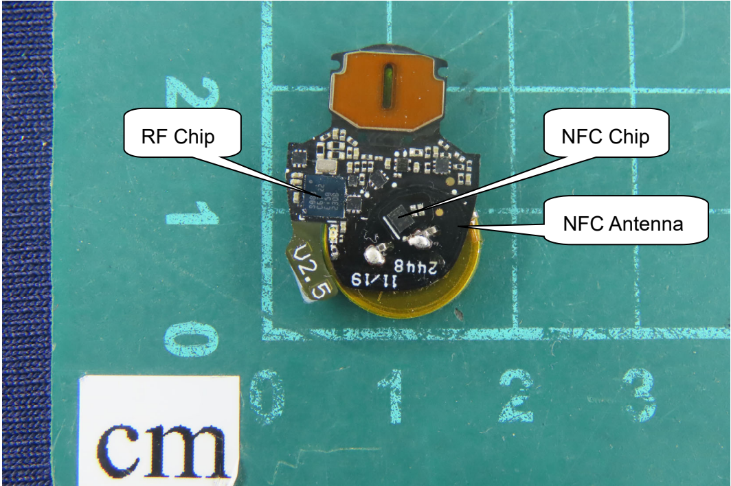
(82) EUT Photo
