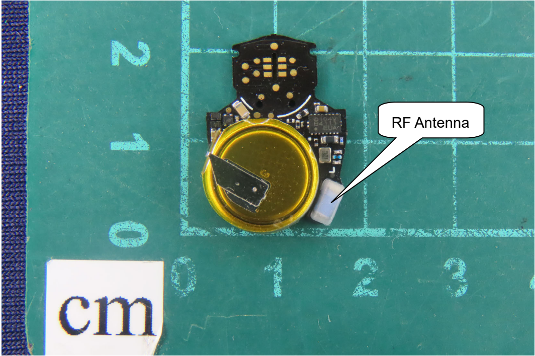
(71) EUT Photo
