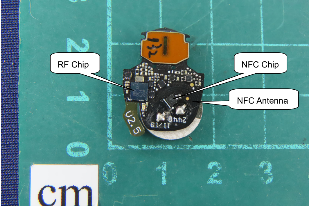
(66) EUT Photo
