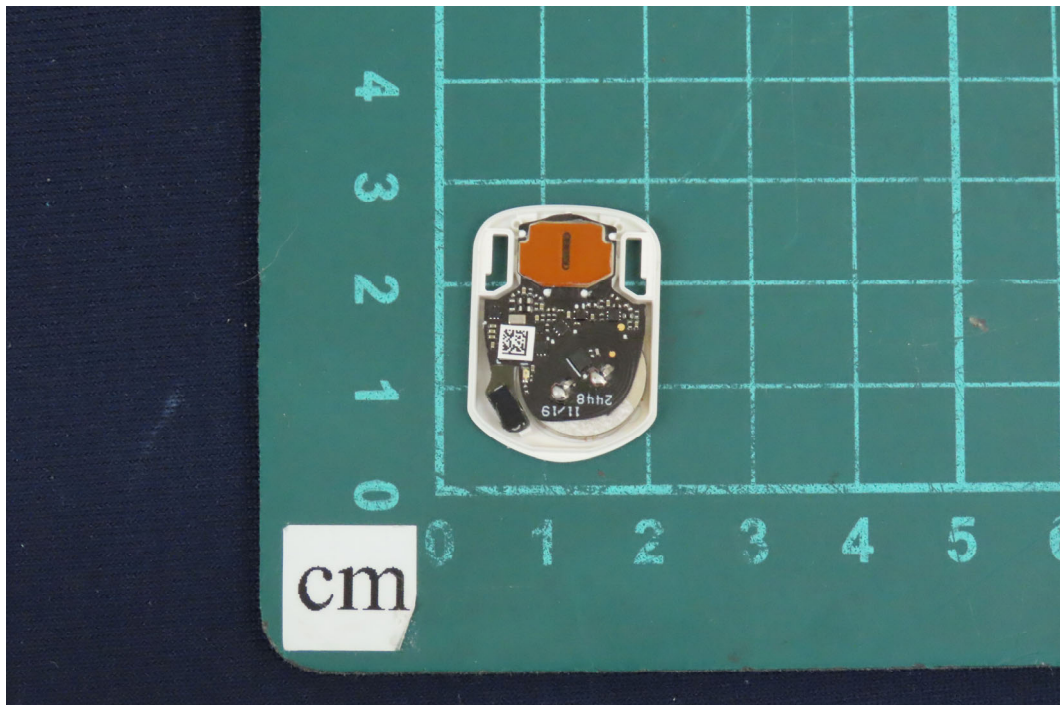
(65) EUT Photo
