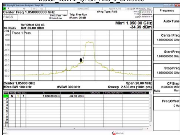
Band2 10MHz QPSK RB6 0 CH18650
