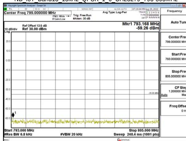
NB IoT Band13 15kHz QPSK 1 0 CH23279 793-805MHz
