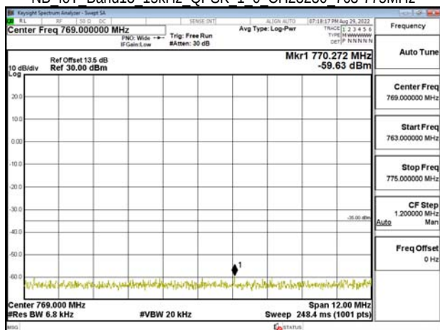
NB IoT Band13 15kHz QPSK 1 0 CH23230 763-775MHz
