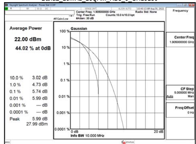
Band2 10MHz 16QAM RB5 0 CH19150
