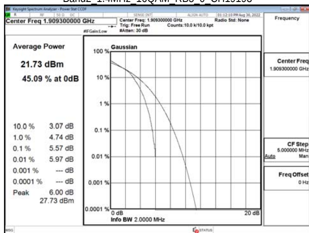
Band2 1.4MHz 16QAM RB5 0 CH19193
