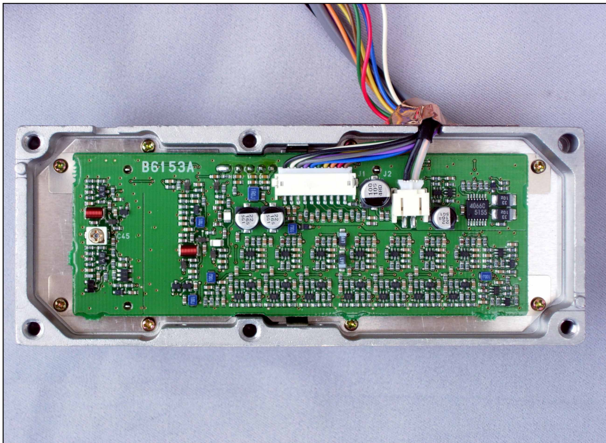
IF Unit
