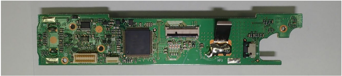
FRONT-D (TOP)
