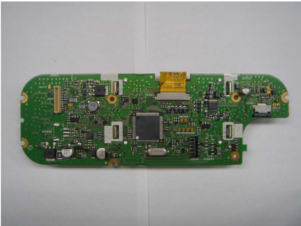
DISPLAY-A UNIT (b o t t o m)
