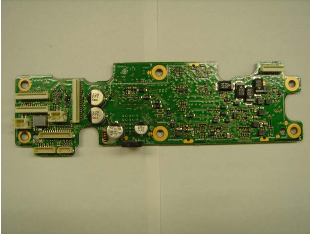
DSP1-A UNIT (t o p)
