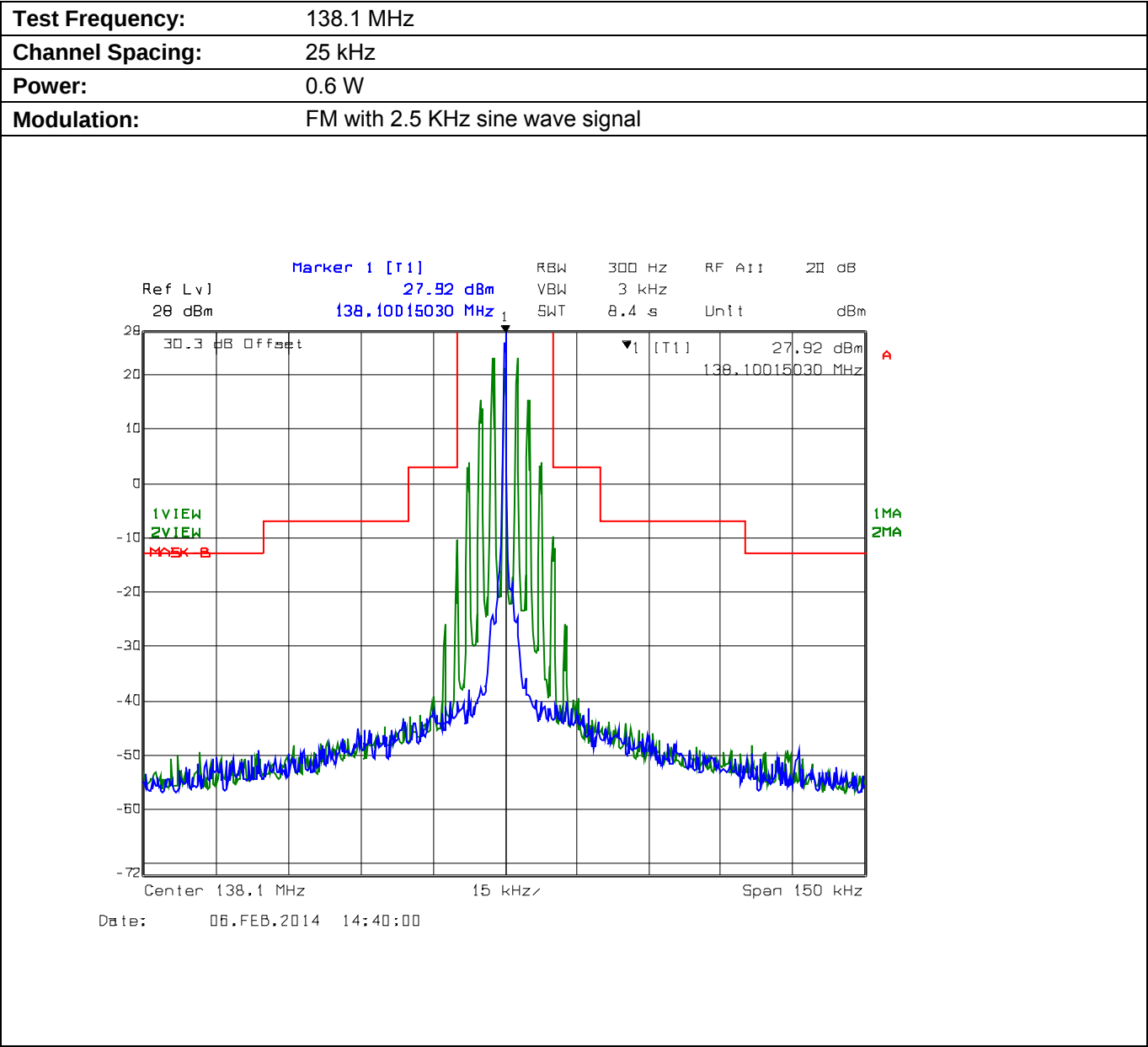
Plot 5.8.4.3.4. Emission Mask B, Low Power
