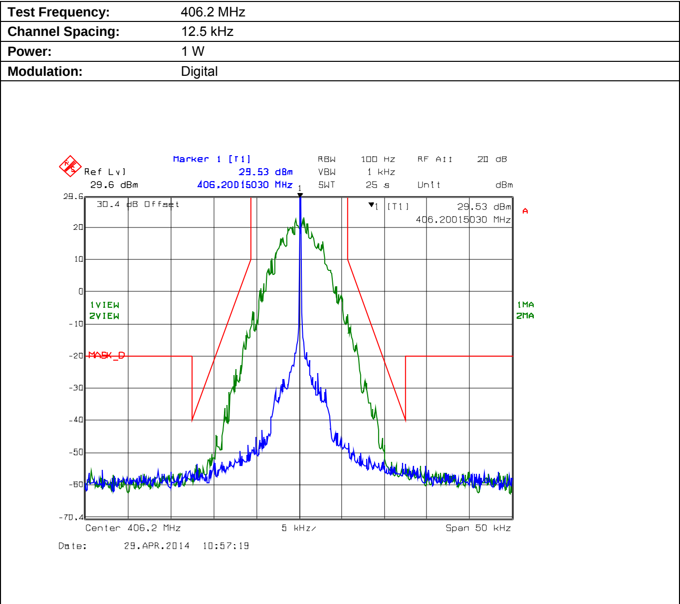
Plot 5.8.4.2.10. Emission Mask D, Low Power
