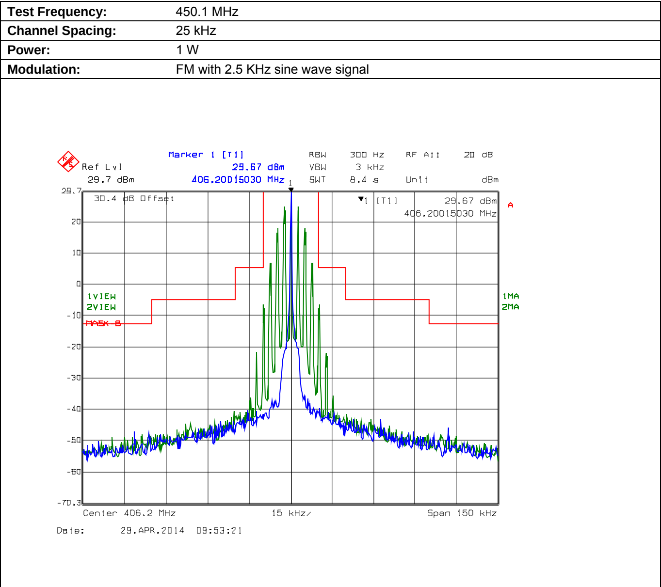
Plot 5.8.4.3.5. Emission Mask B, Low Power
