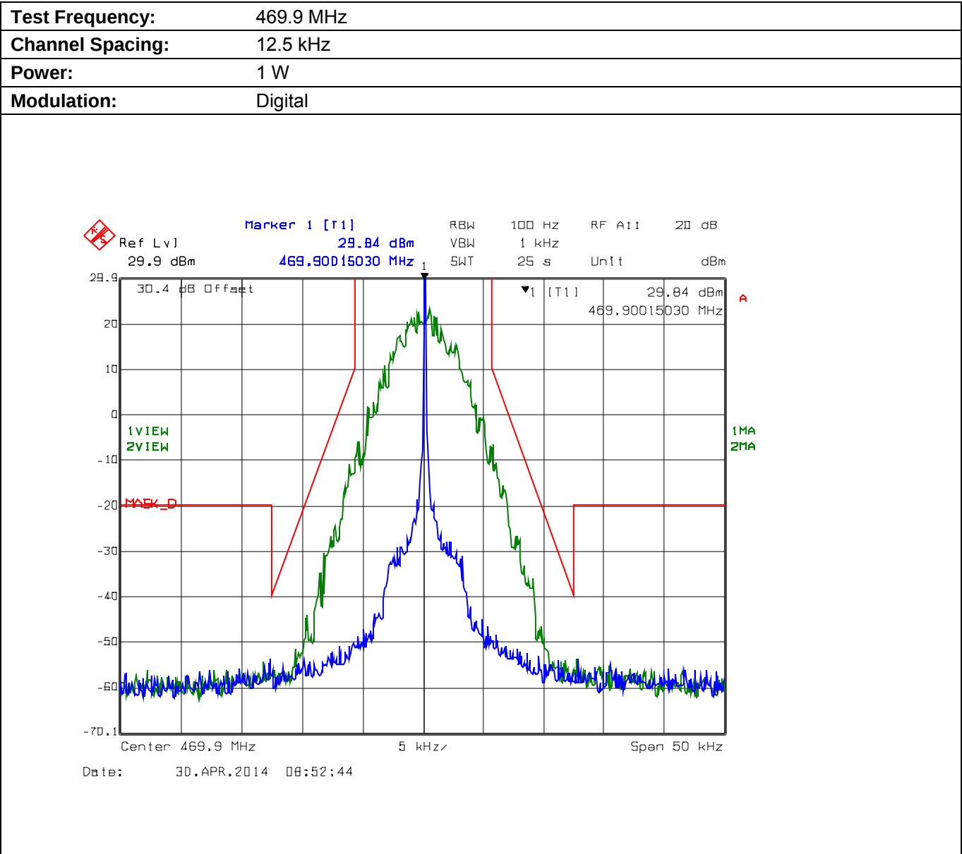
Plot 5.8.4.2.12. Emission Mask D, Low Power
