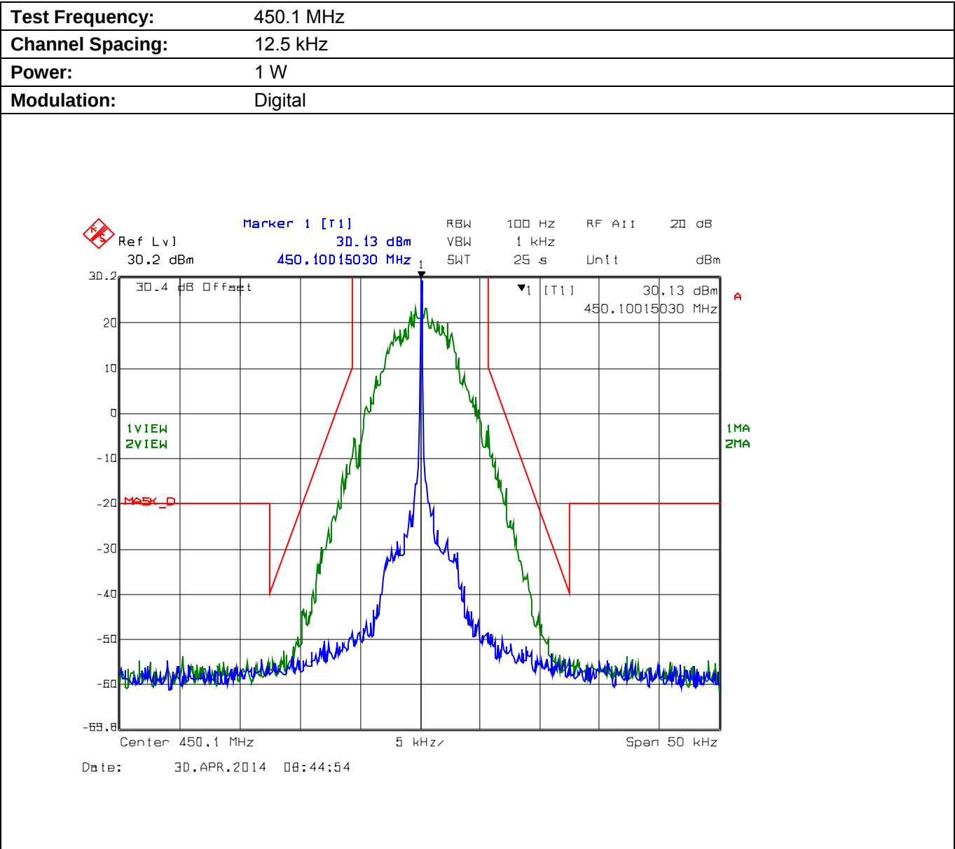
Plot 5.8.4.2.11. Emission Mask D, Low Power
