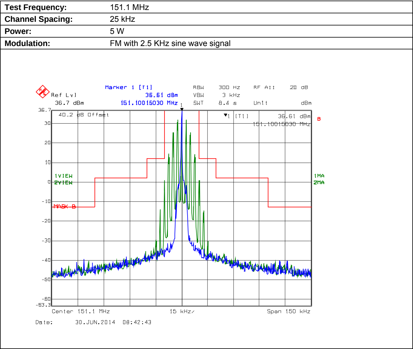
Plot 5.8.4.3.5. Emission Mask B, Low Power
