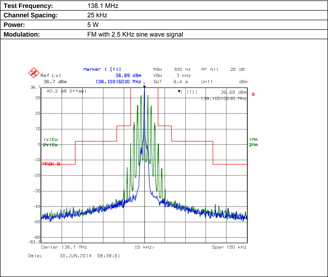
Plot 5.8.4.3.4. Emission Mask B, Low Power
