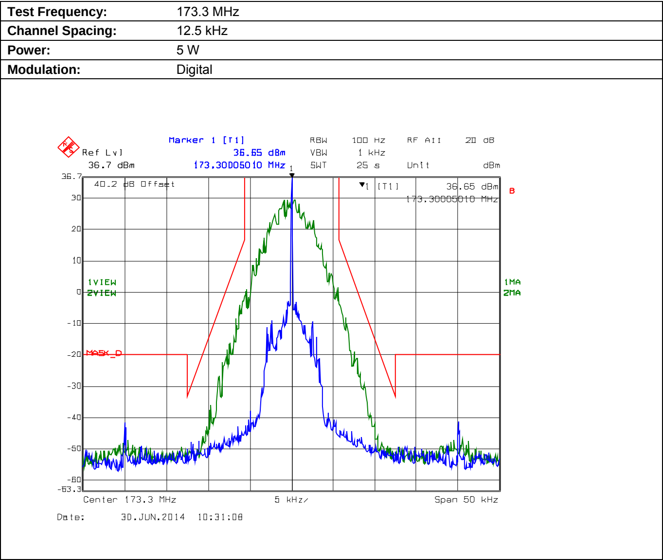
Plot 5.8.4.2.12. Emission Mask D, Low Power
