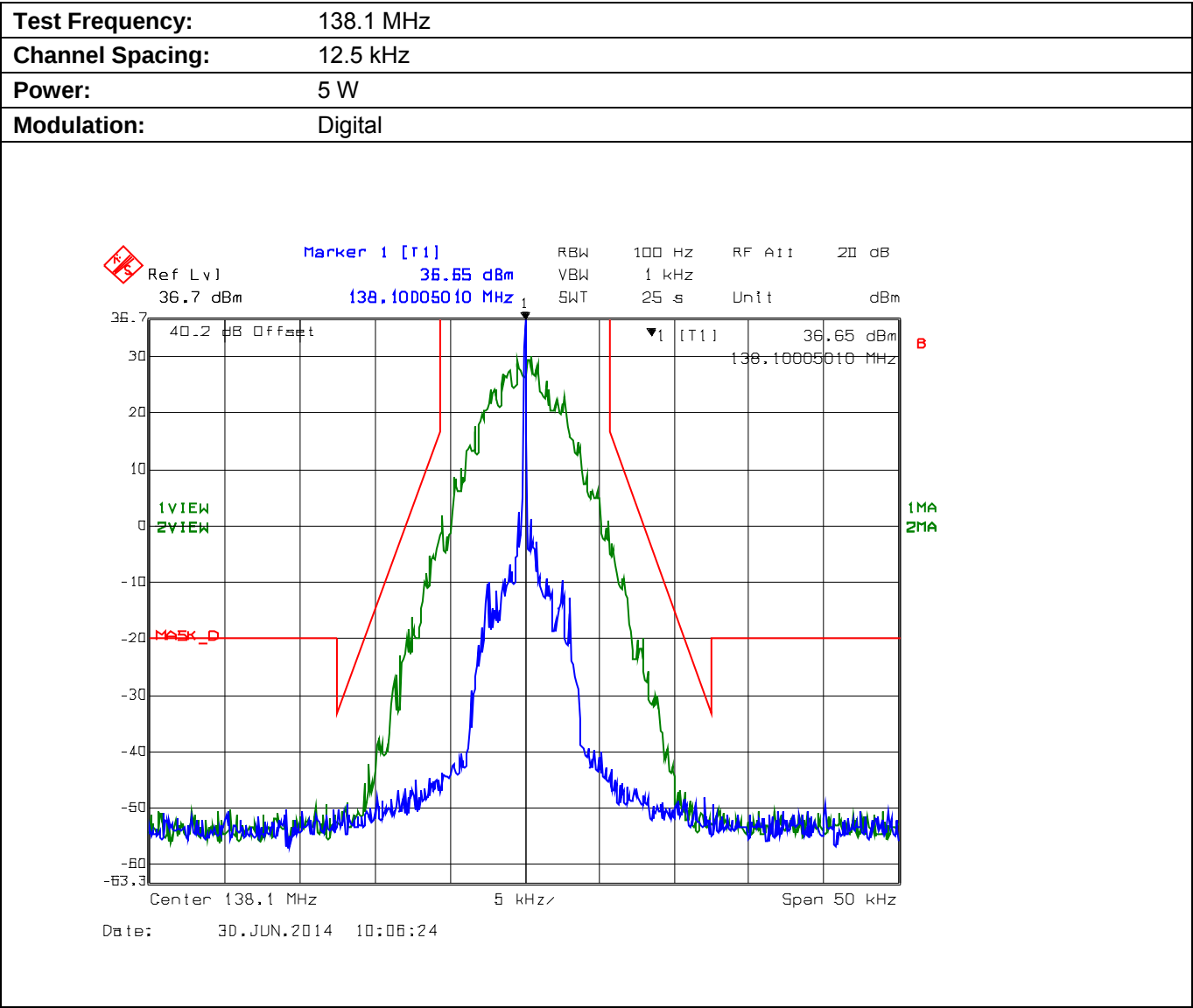
Plot 5.8.4.2.10. Emission Mask D, Low Power
