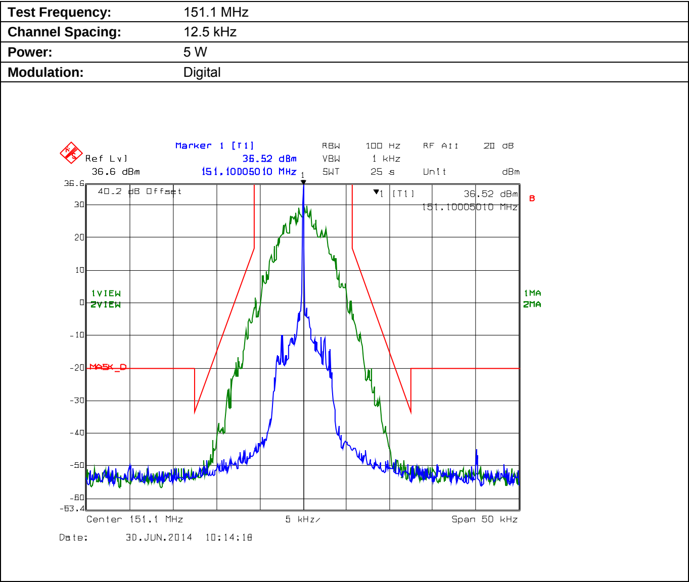
Plot 5.8.4.2.11. Emission Mask D, Low Power
