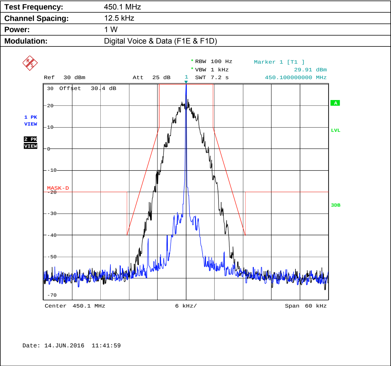
Plot 5.8.4.2.11. Emission Mask D, Low Power
