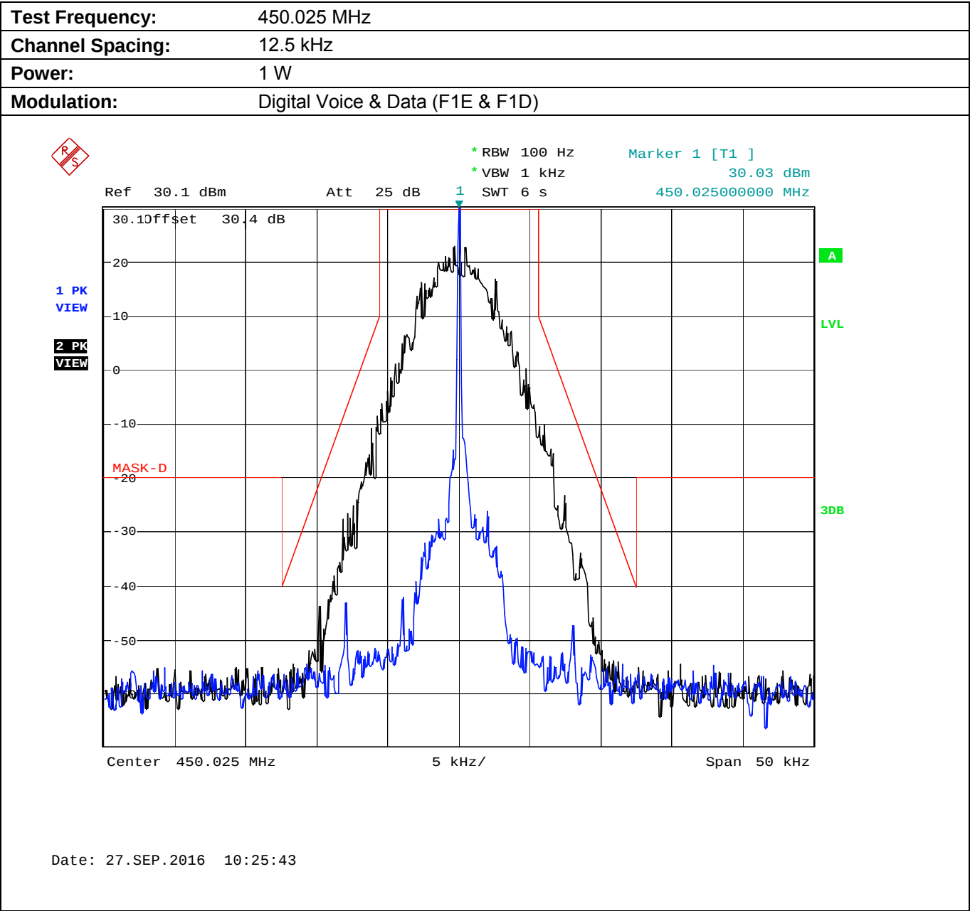
Plot 5.8.4.2.10. Emission Mask D, Low Power
