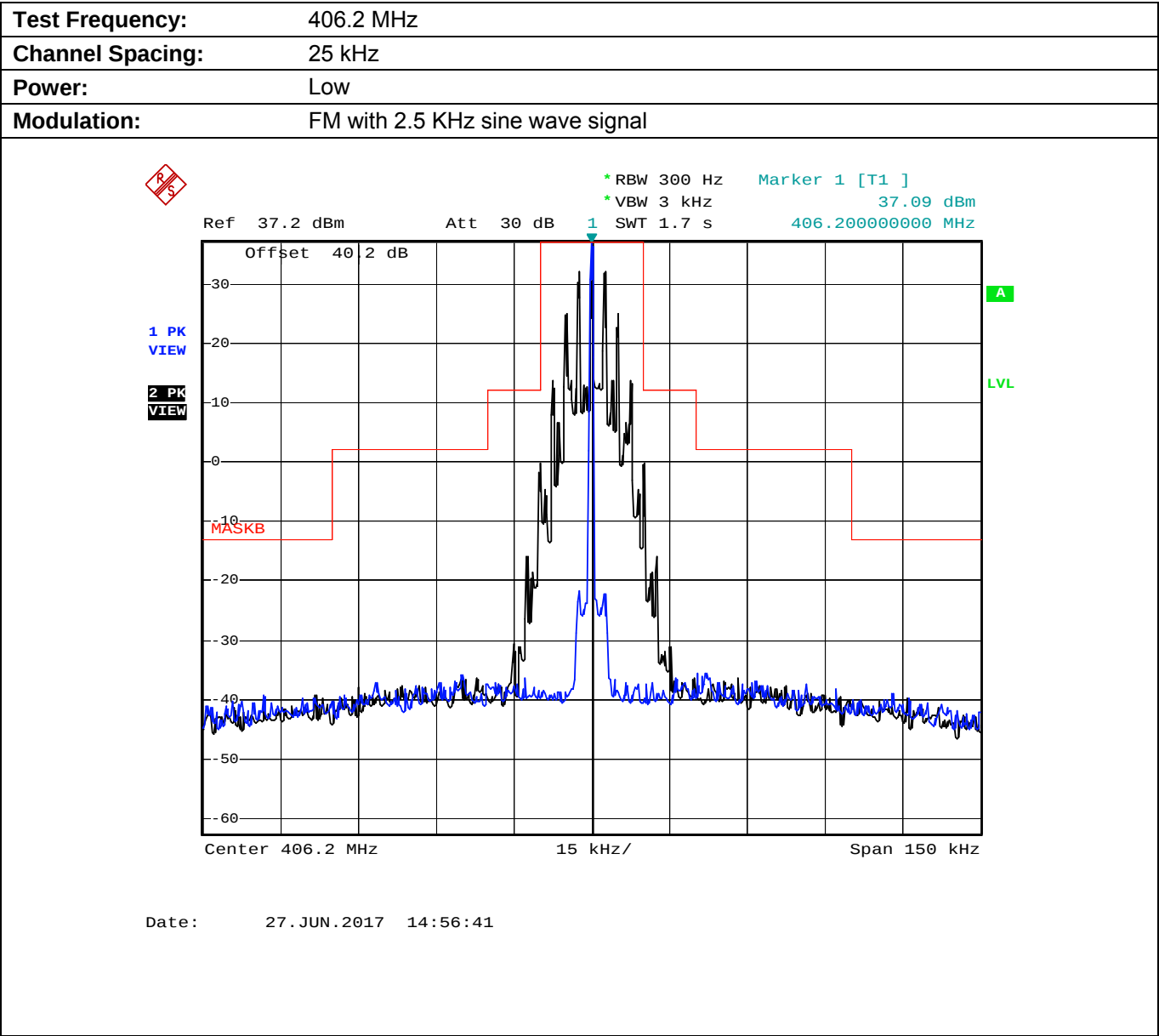
Plot 5.8.4.3.4. Emission Mask B, Low Power
