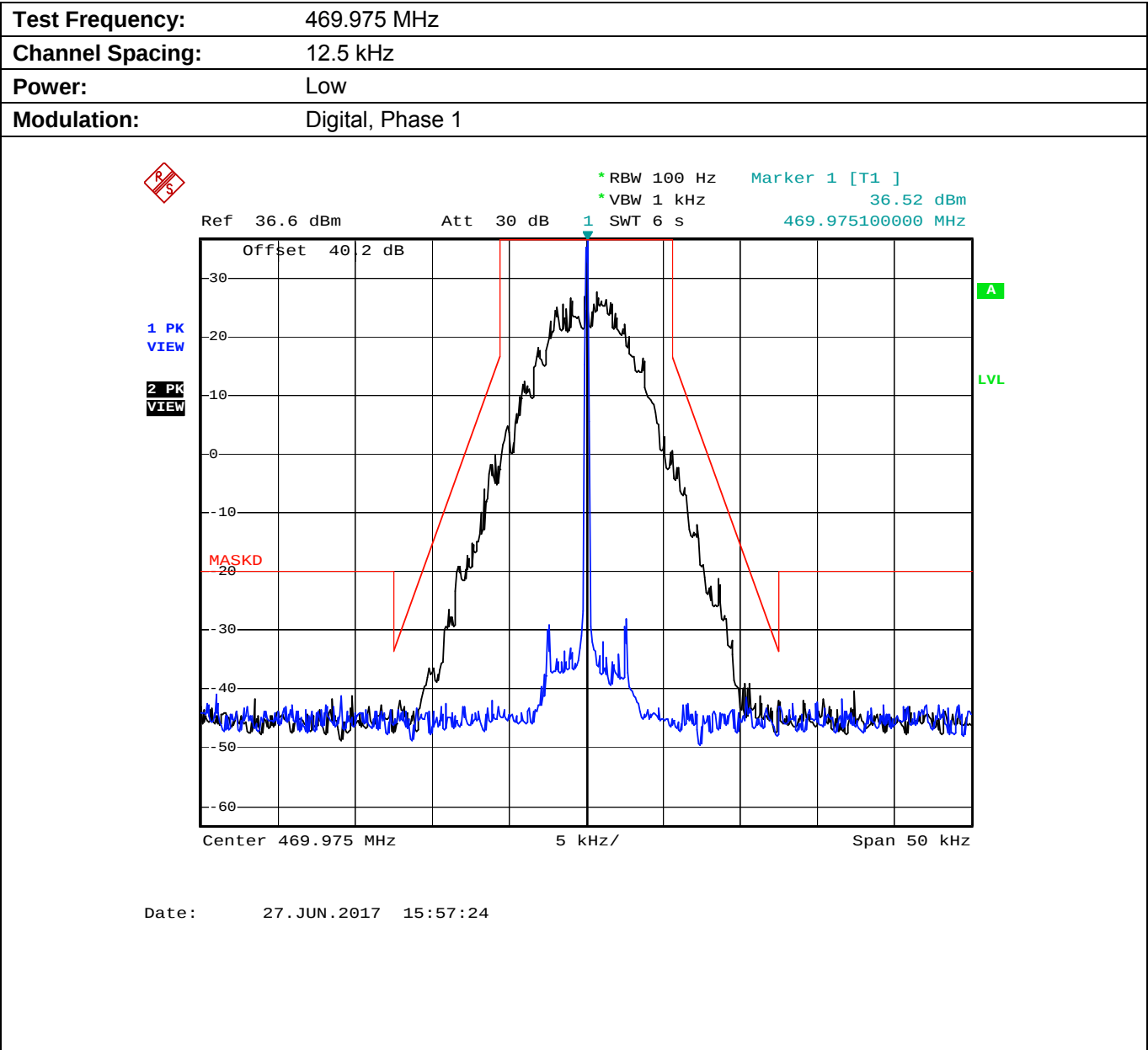
Plot 5.8.4.2.12. Emission Mask D, Low Power
