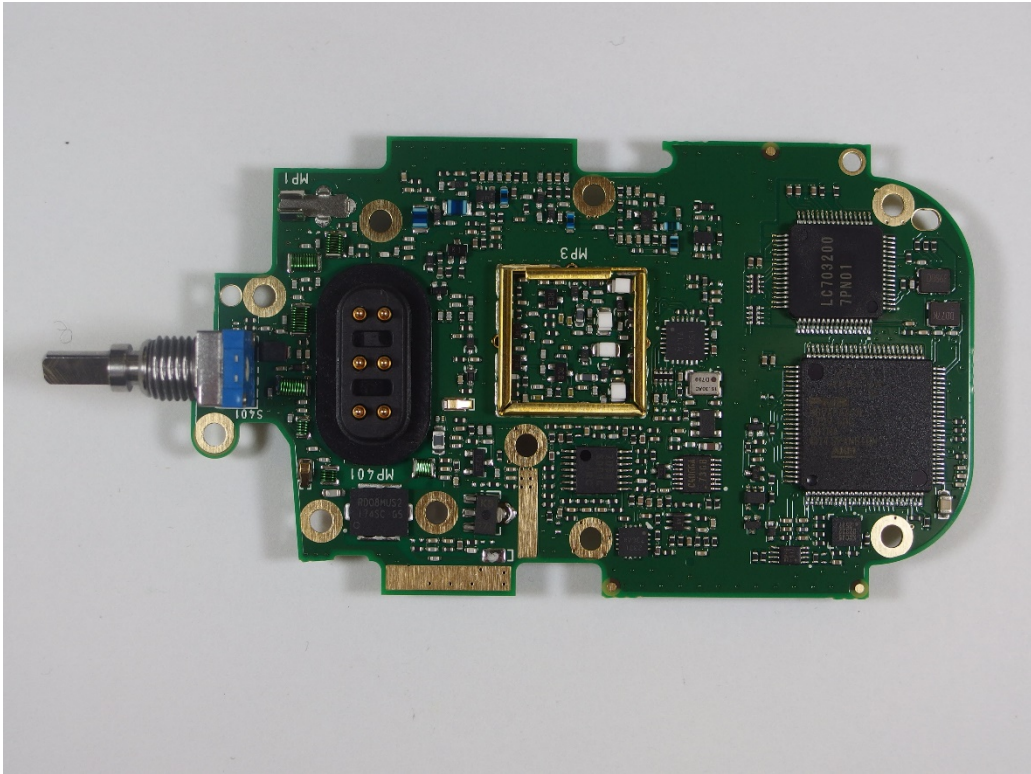
PCB_MAIN_B
