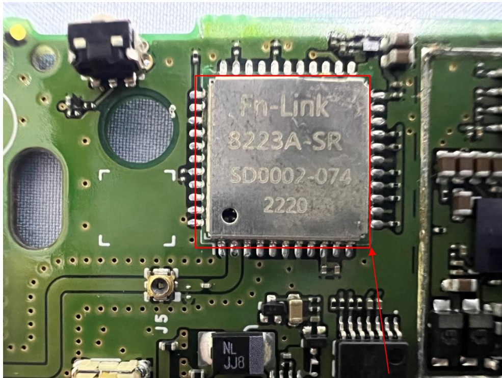
WIFI Module
