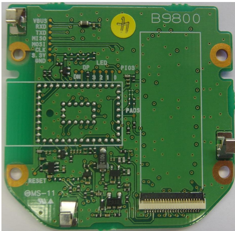
FRONT-1_B_non Bluetooth Ver.
