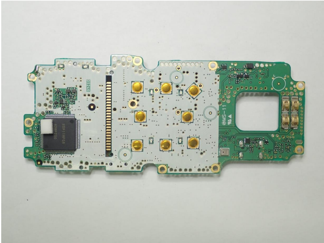
PCB_MAIN-A
