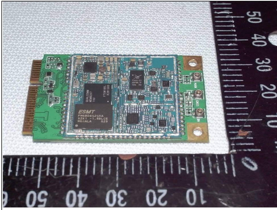
PCB-2
