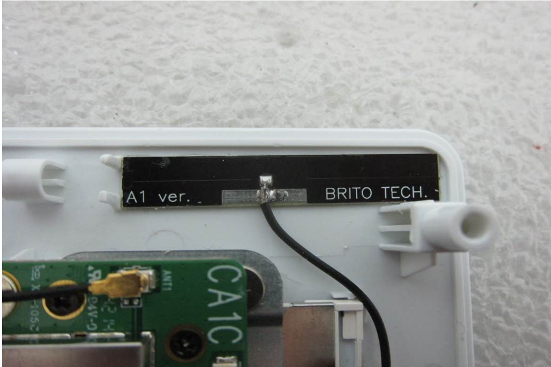
EUT 8 Zigbee Antenna
