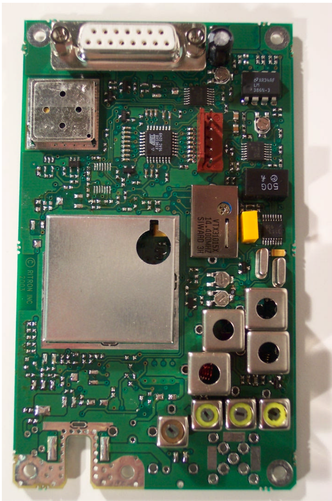
DR-142 PCB top
