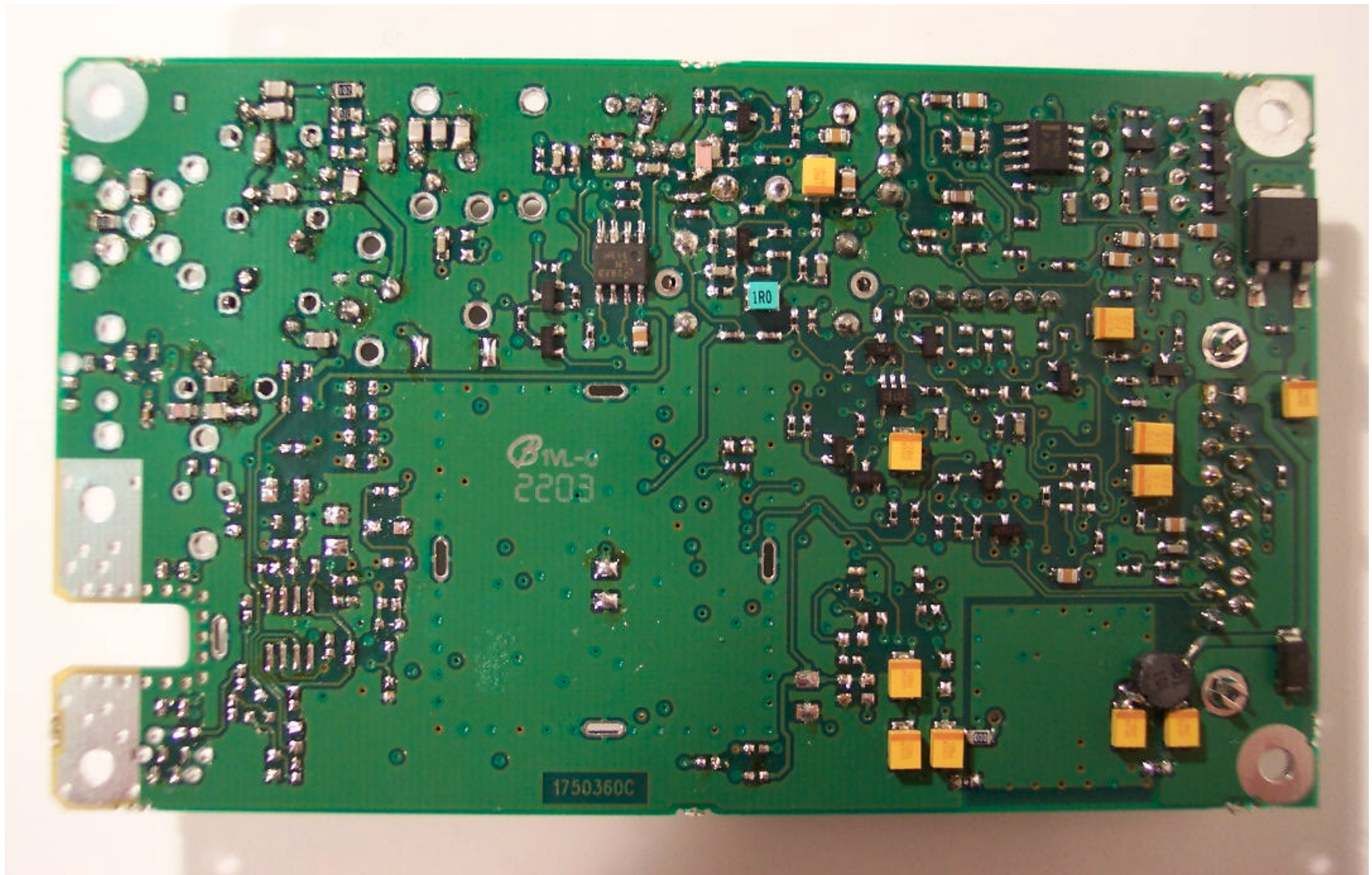
DR-142 PCB bottom
