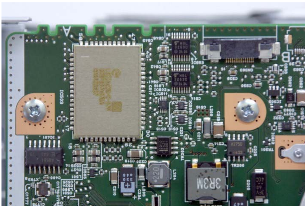
RF Module
