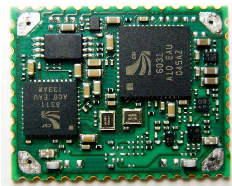
<半田付けを取り、シールド外した状態(without Shield)>
