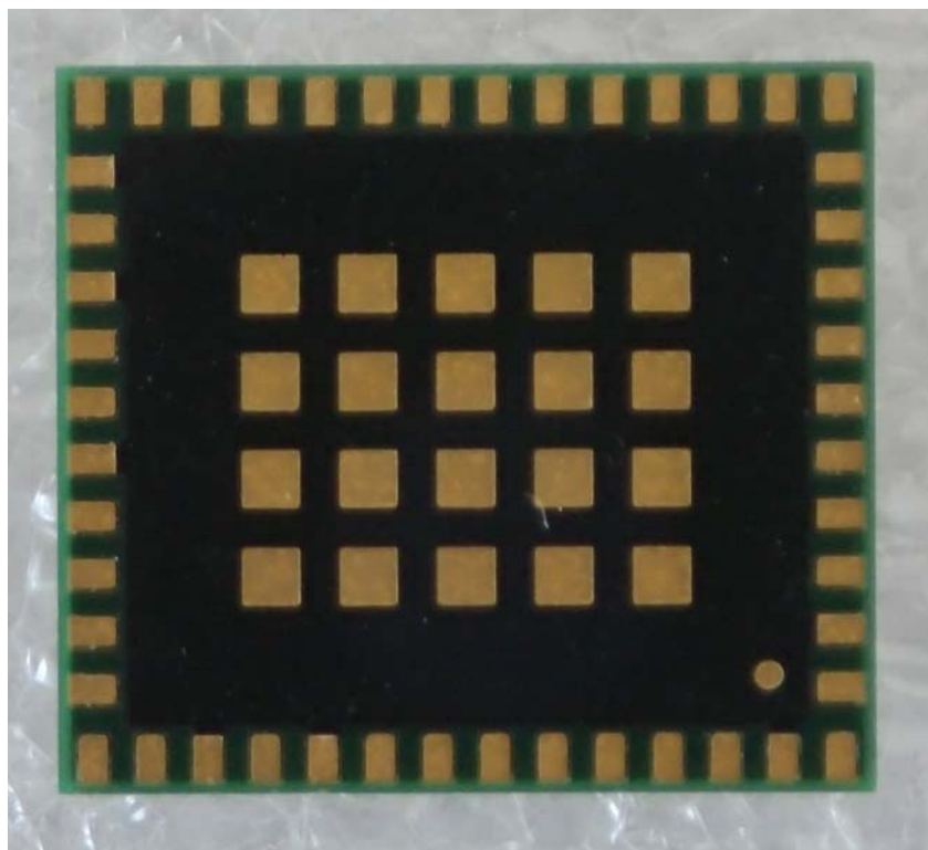
WLAN BT Combo Module
