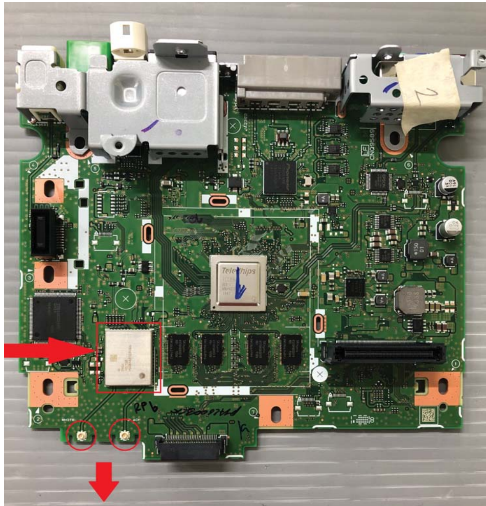
RF Module
