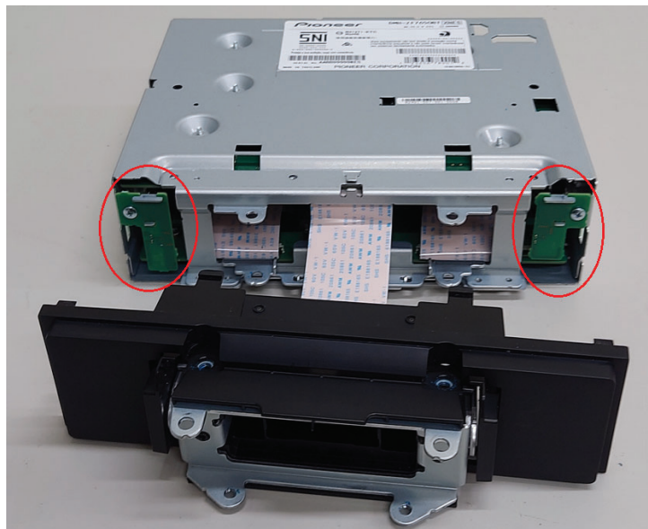
Wi-Fi Antenna (5GHz)
