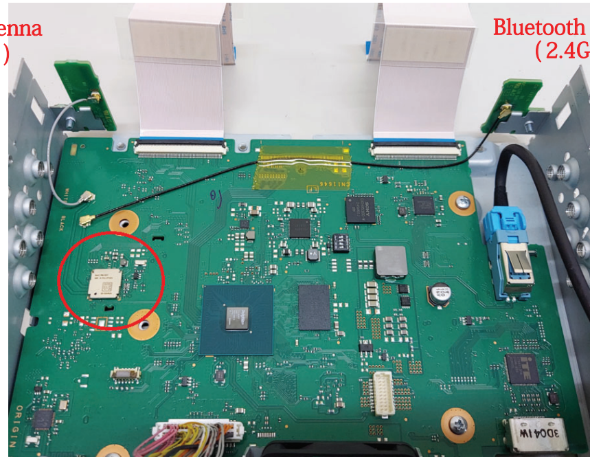
RF Module
