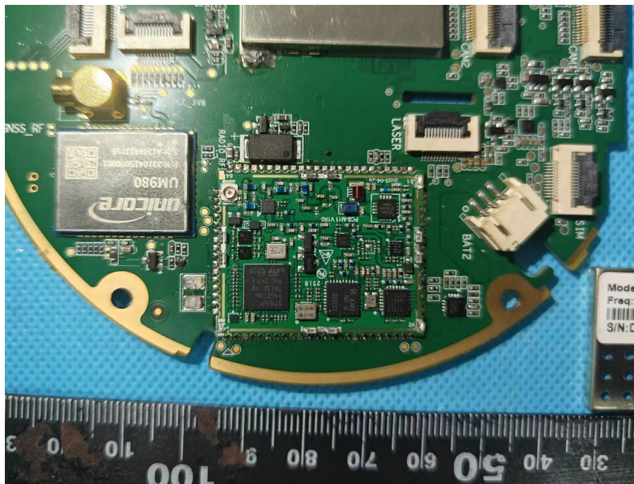
Radio module
