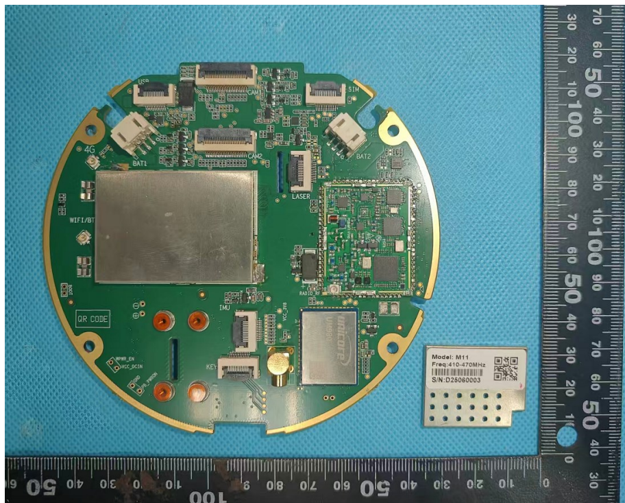
Radio module
