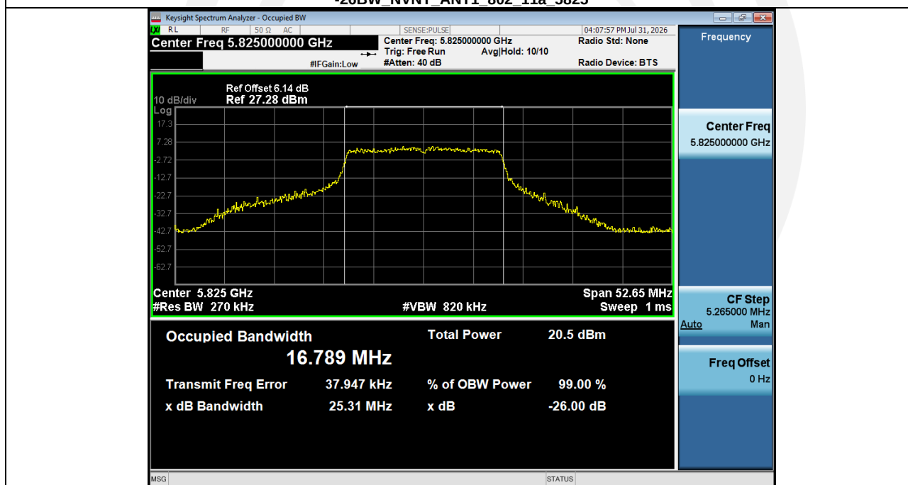
-26BW NVNT ANT1 802 11a 5825
