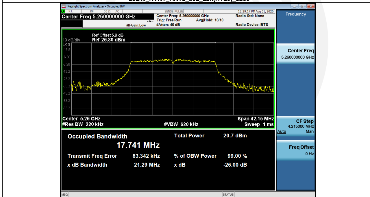
-26BW NVNT ANT1 802 11n(HT20) 5260
