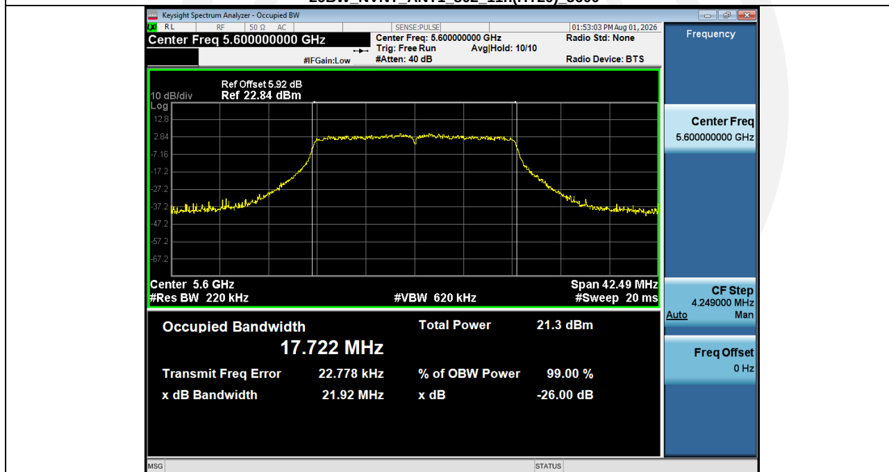
-26BW NVNT ANT1 802 11n(HT20) 5600
