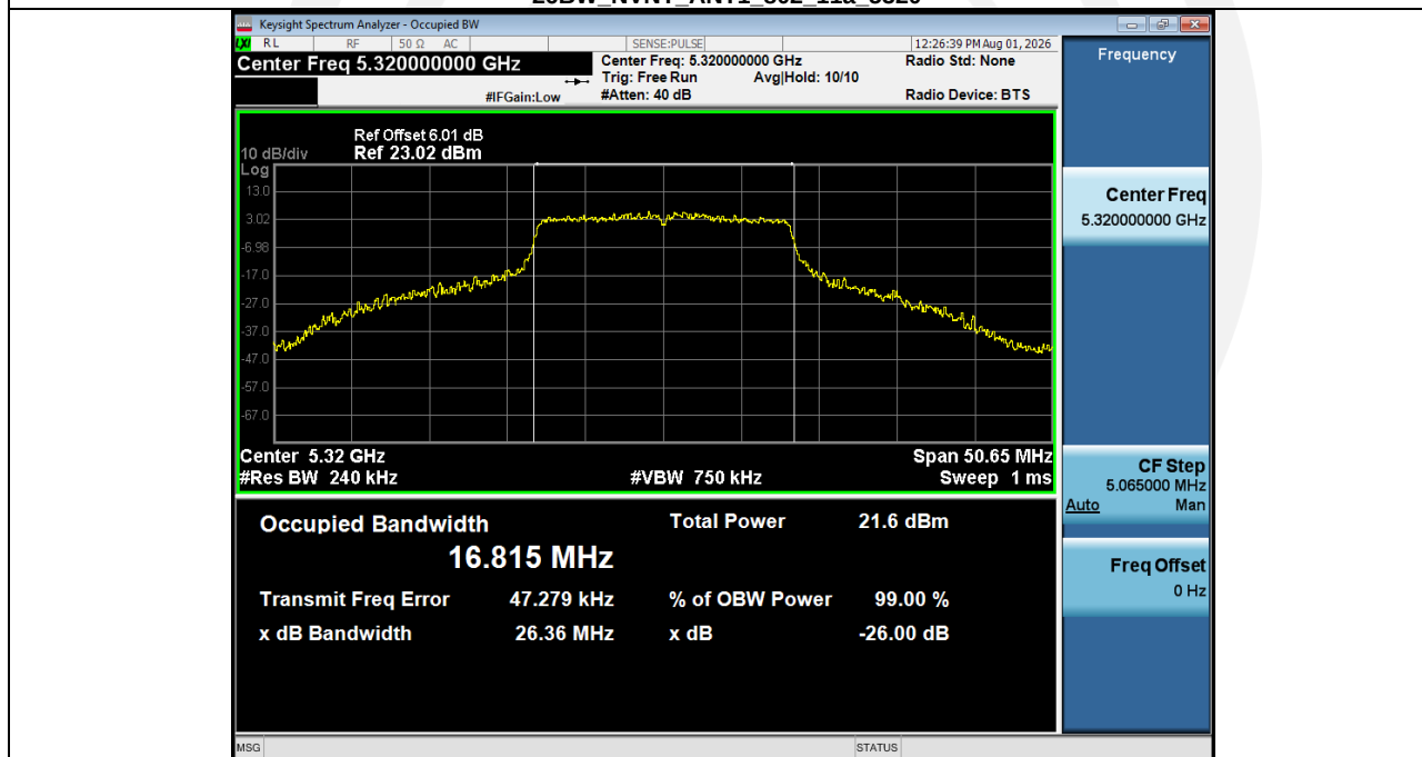
-26BW NVNT ANT1 802 11a 5320
