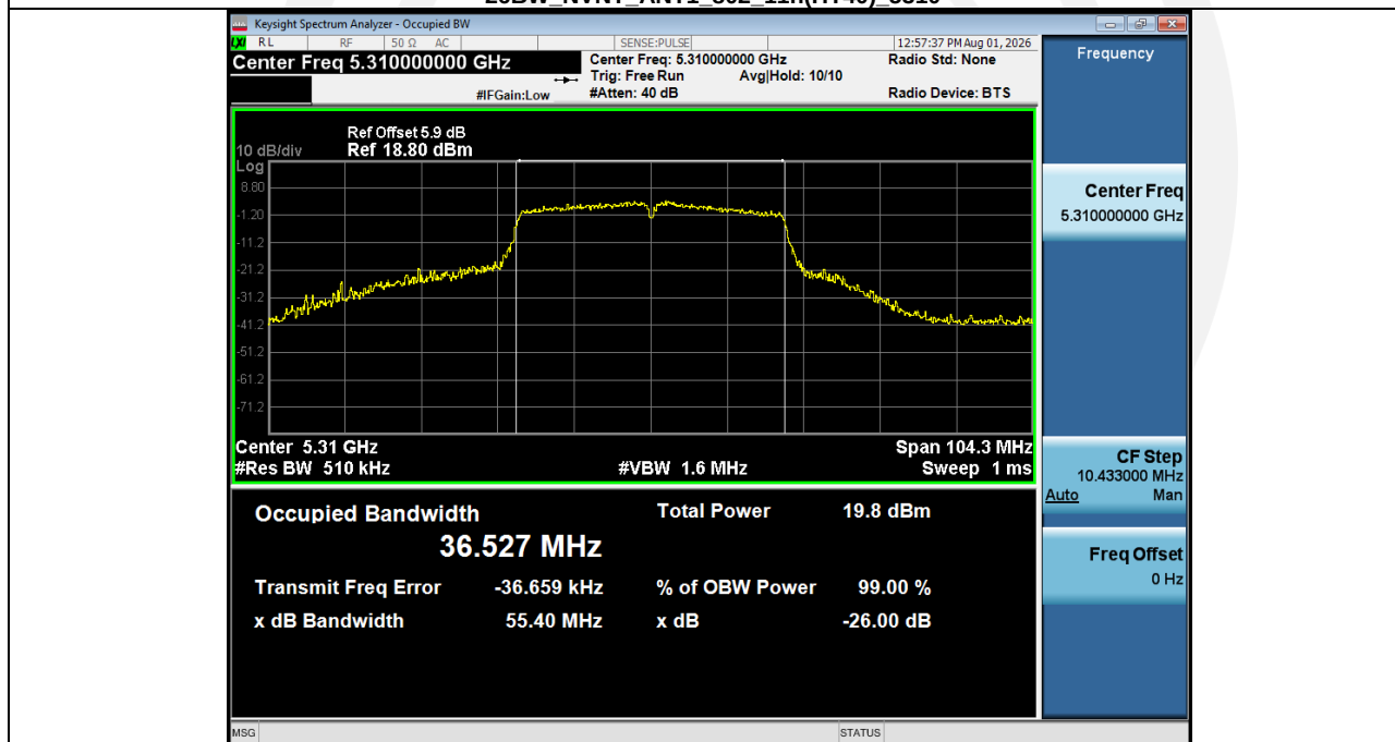
-26BW NVNT ANT1 802 11n(HT40) 5310
