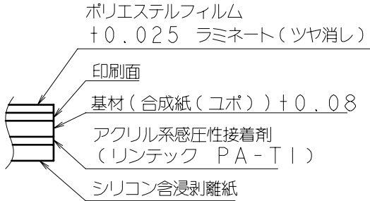
材料構成図
