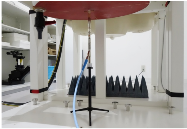
D2450V2
