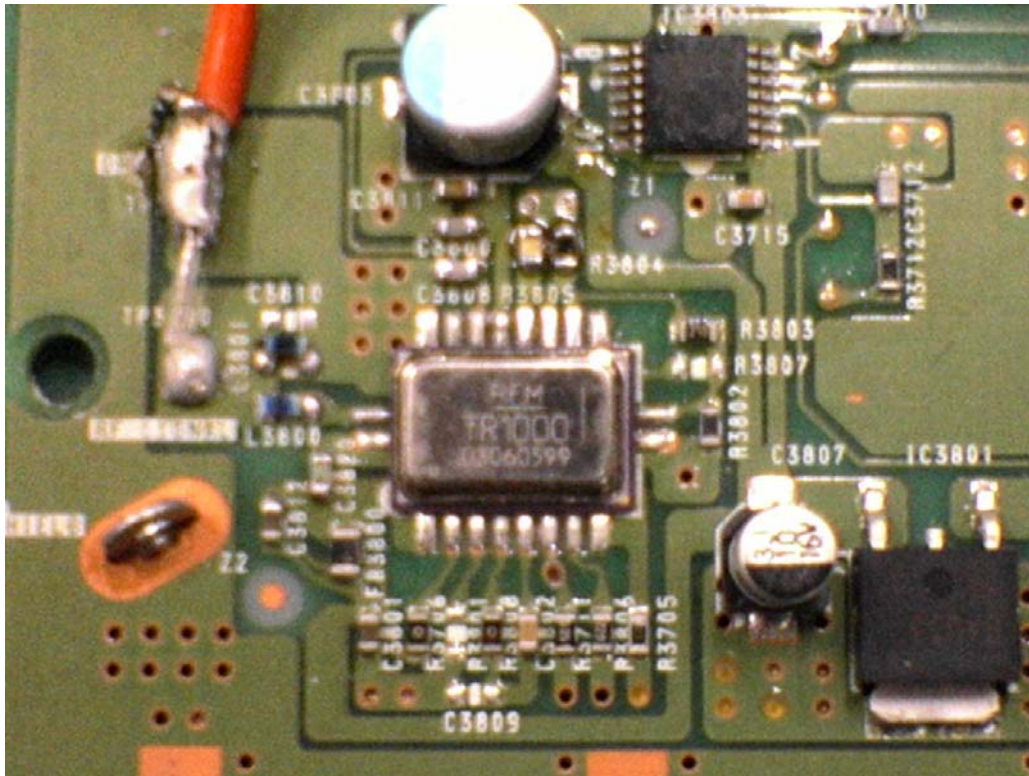
Module (enlargement)
