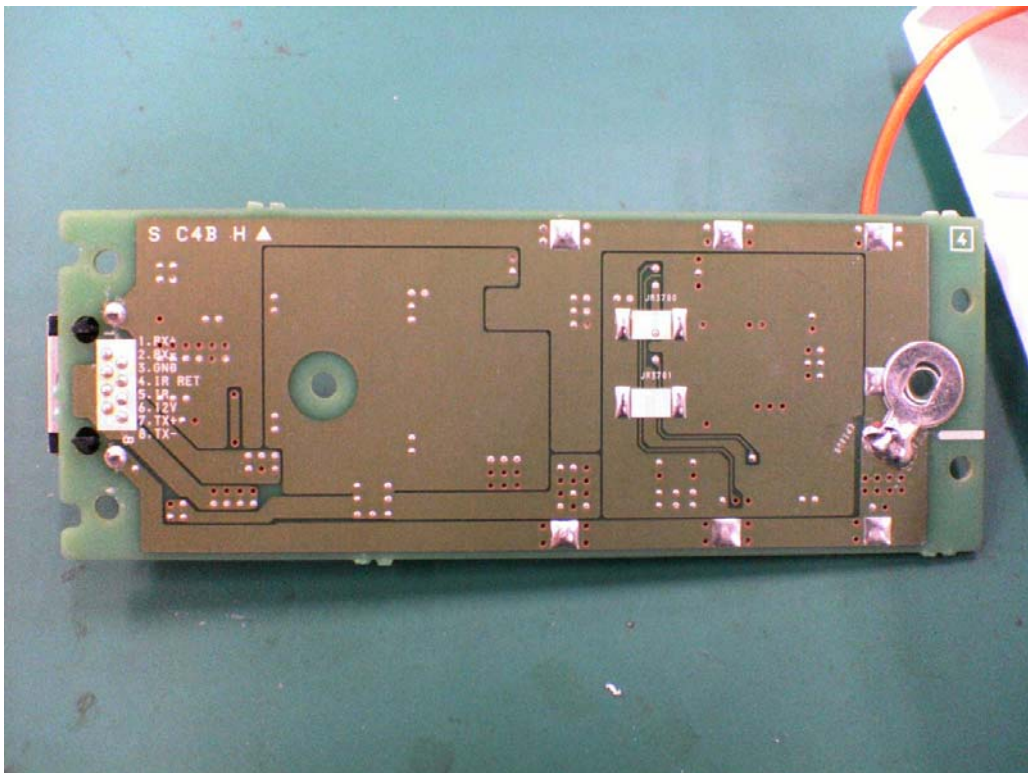
Module (Bottom)
