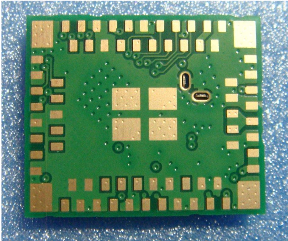
Front-end Bottom
