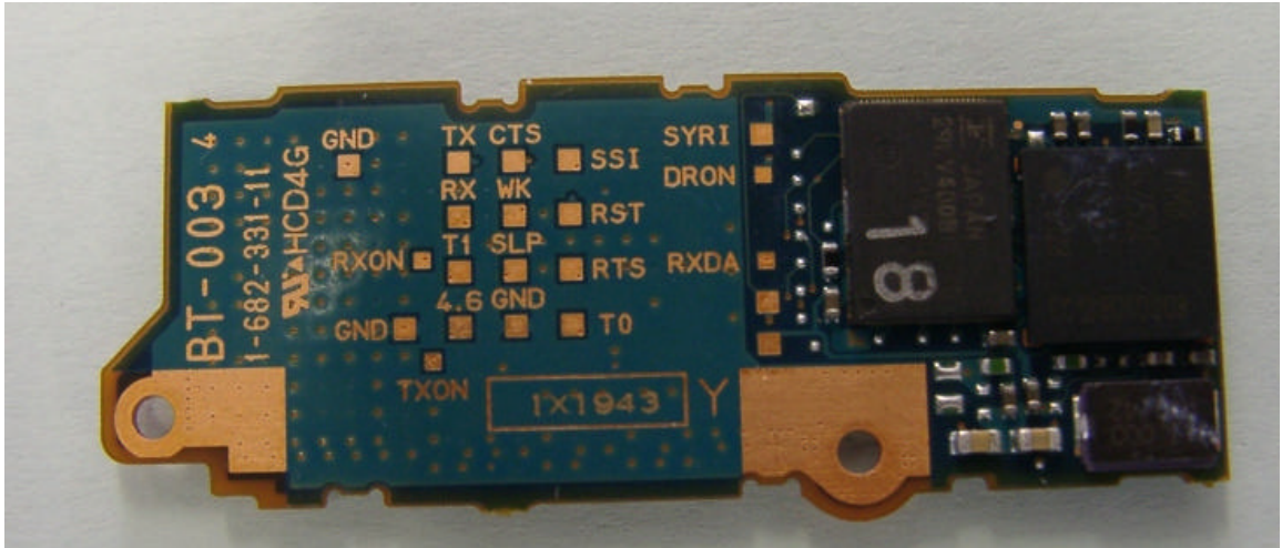
BLUETOOTH MODULE BOTTOM
