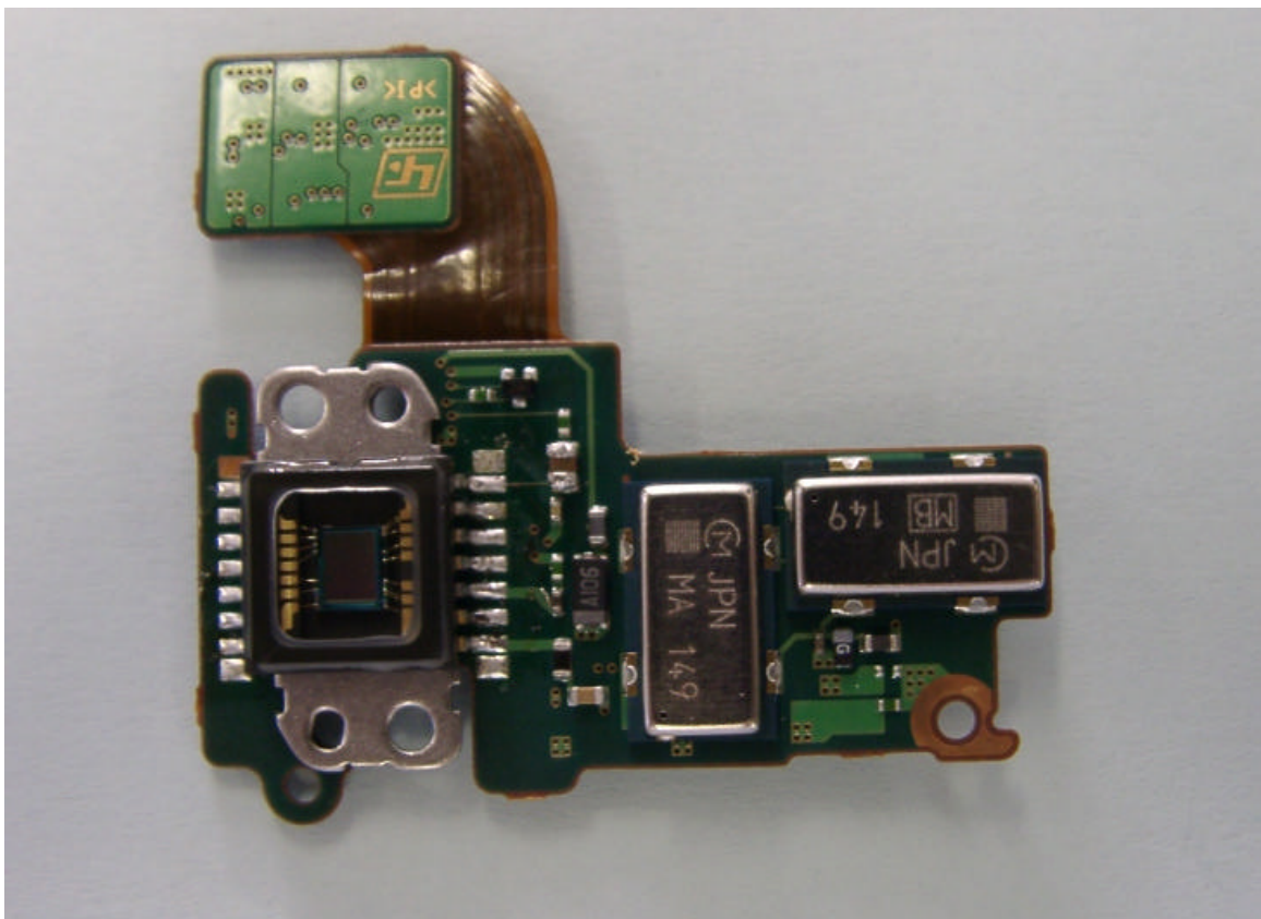
CCD TOP
