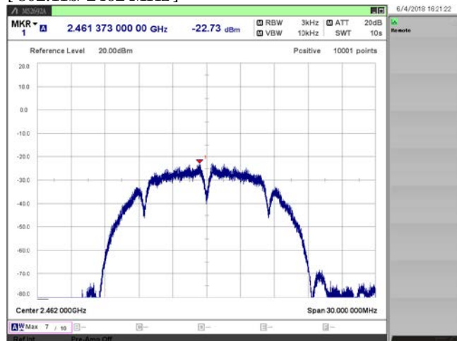
[ 802.11b/ 2462 MHz ]
