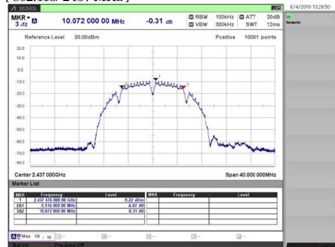
[ 802.11b/ 2437 MHz ]
