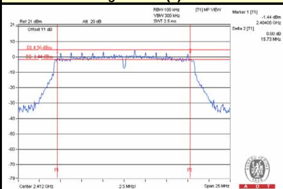
802.11g / Chain (1) : CH1
