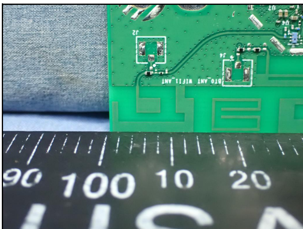
Antenna_Wifi 1
