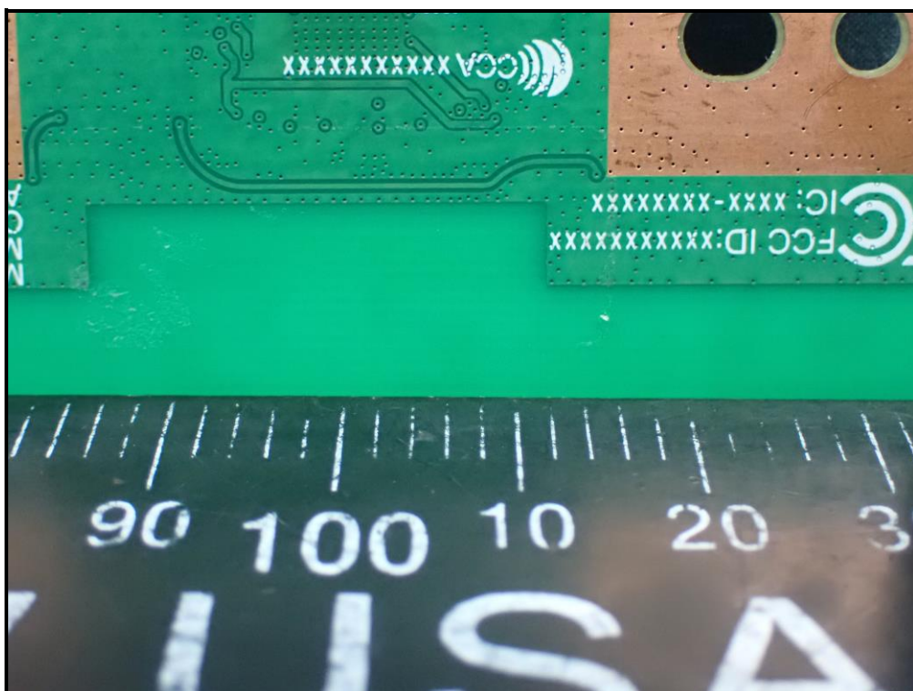
Antenna_BT 1
