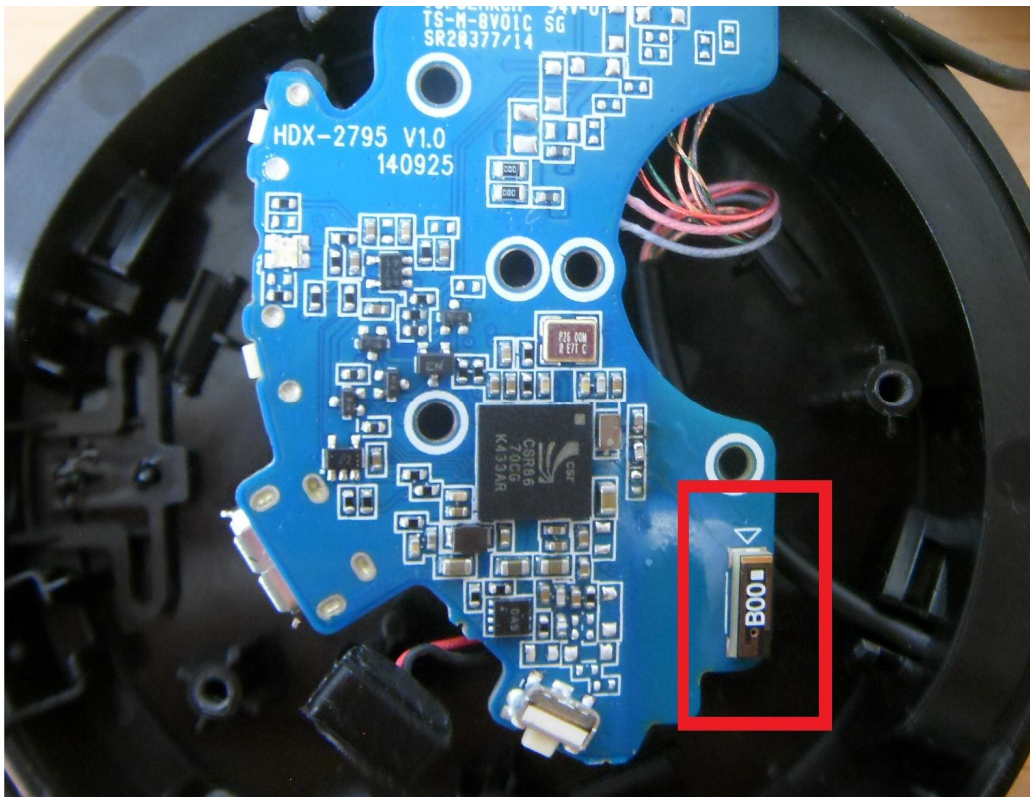
Antenna
