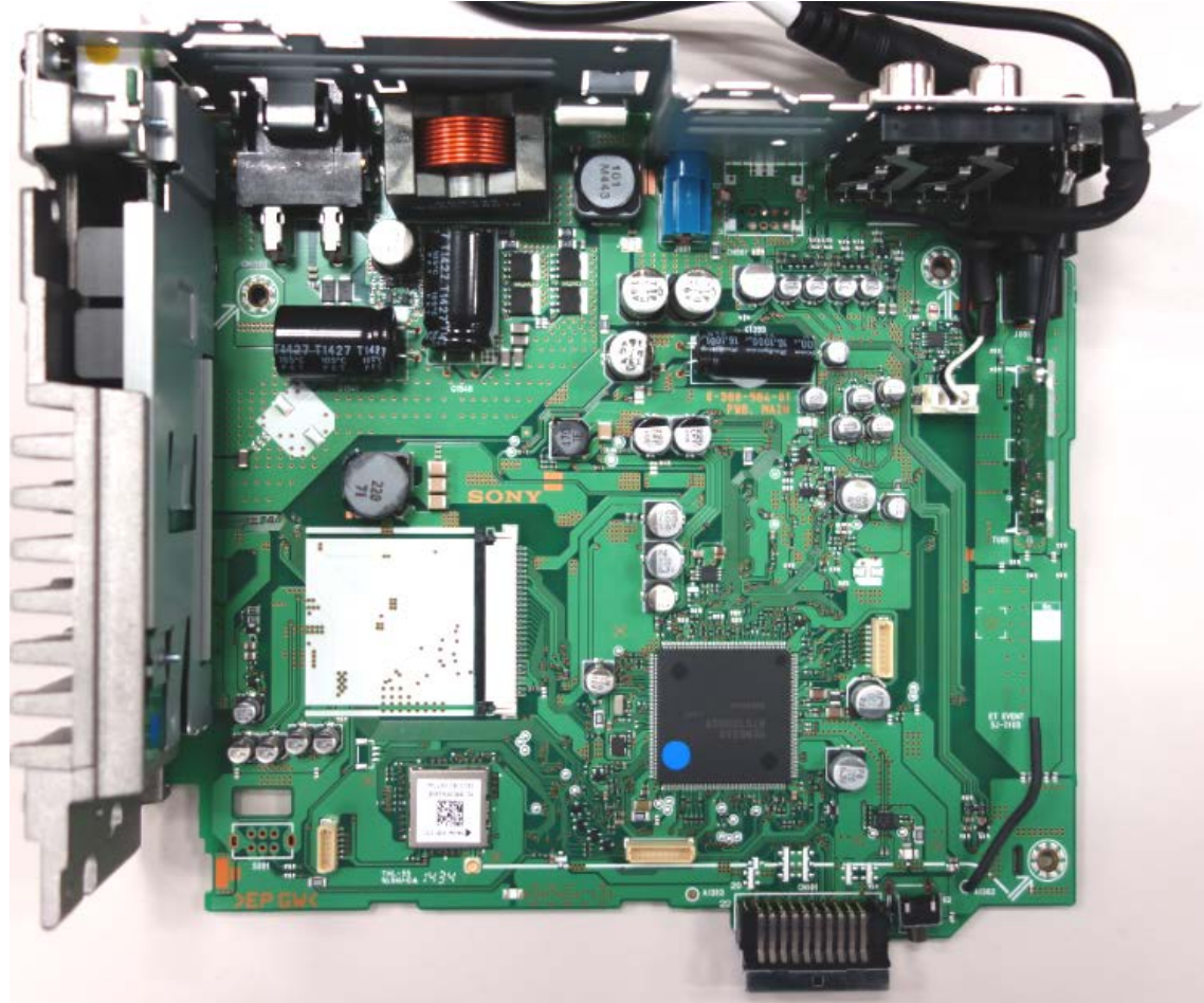
◁MAIN PWB A-side▷
