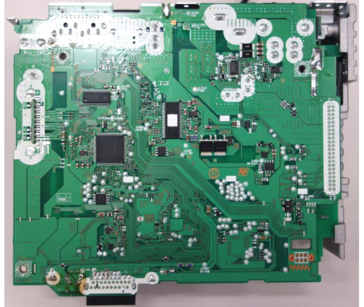
◁MAIN PWB B-side▷
