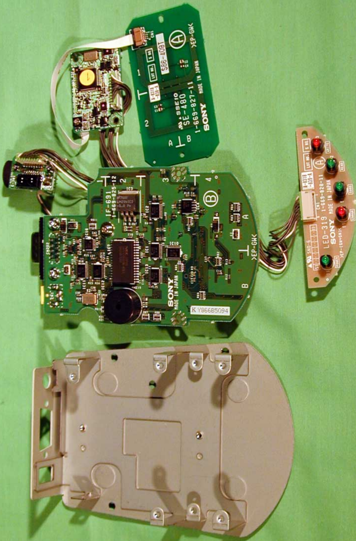
Model: MLU-100A
