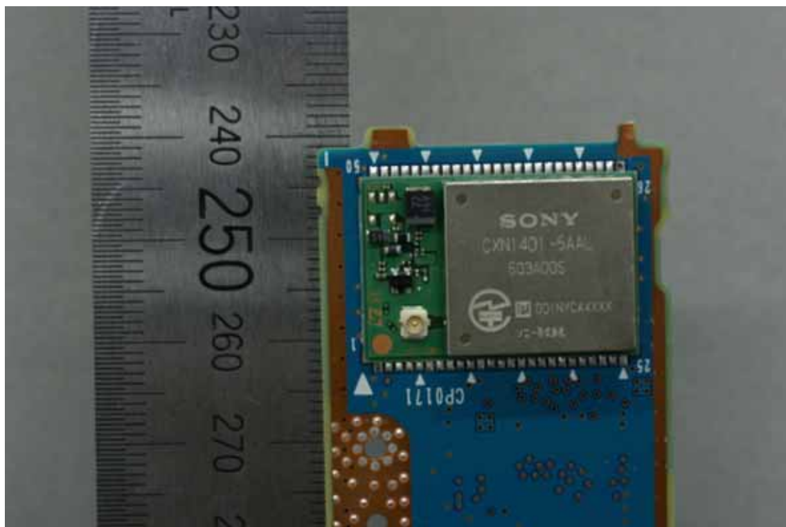
BT Module
