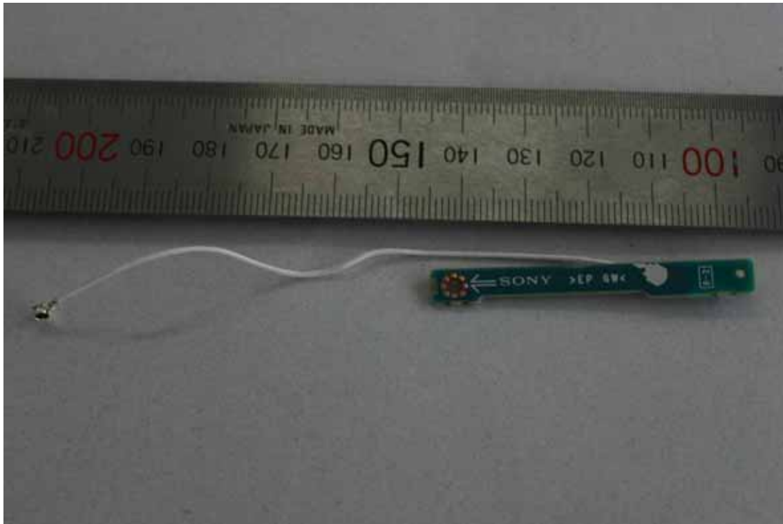
BT ANT
