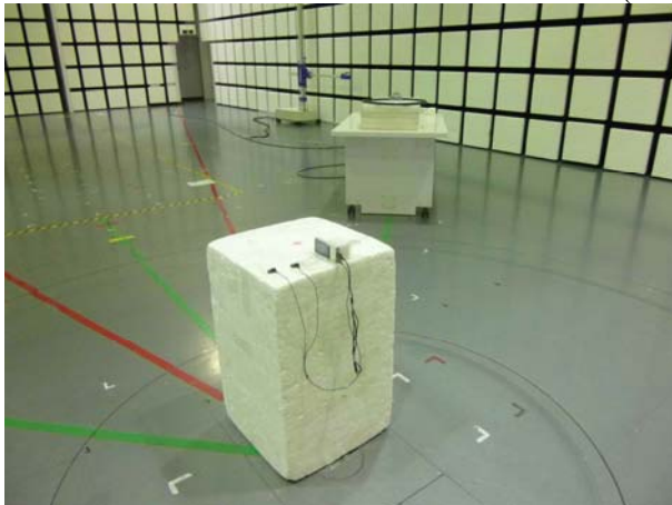
Rear (30-1000MHz)
