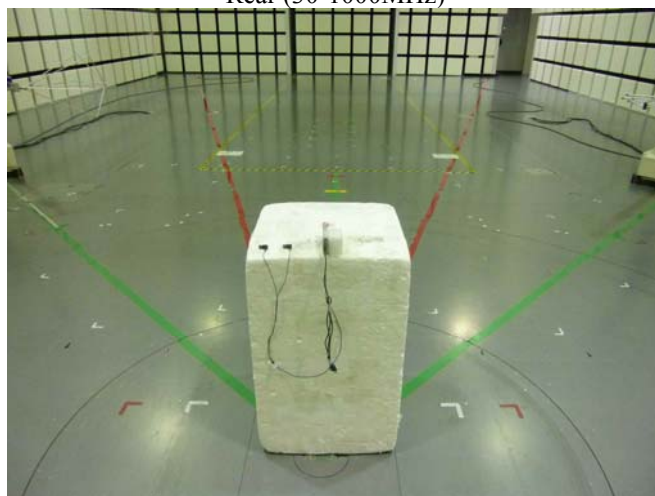
Rear (30-1000MHz)
