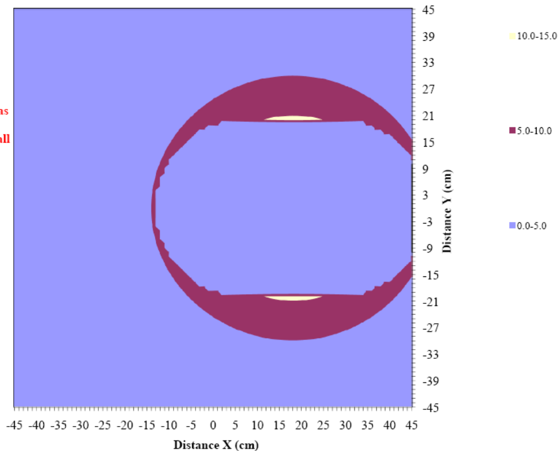
% MPE Contour
