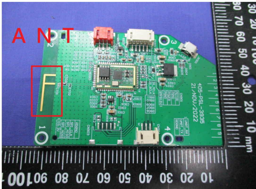
Antenna
