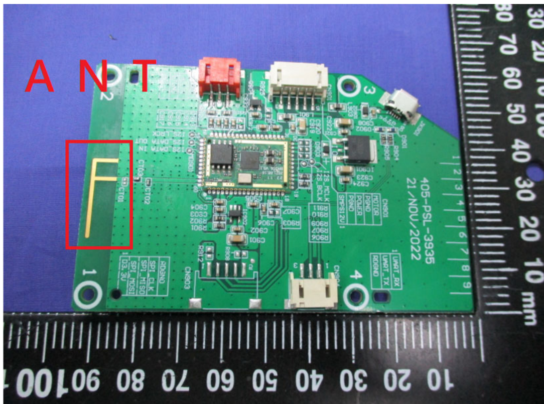
Antenna
