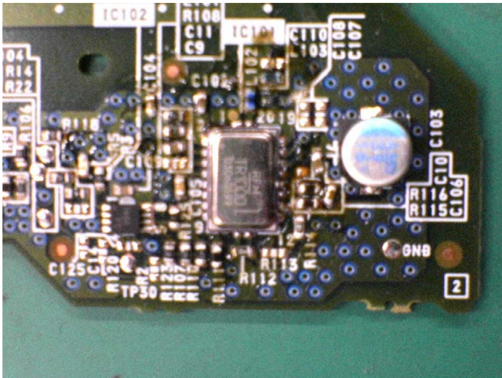
RF Module (Enlargement 1)
