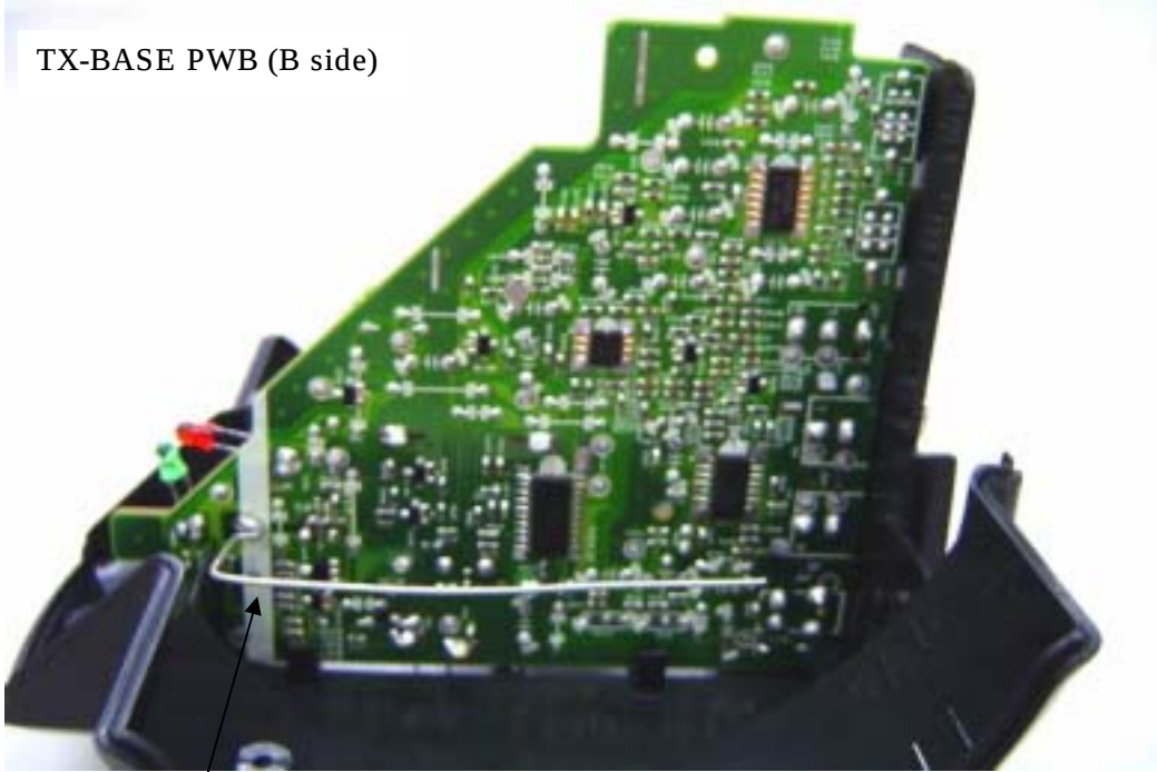
Antenna
