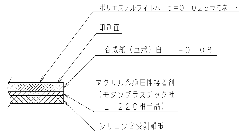
材料構成図
