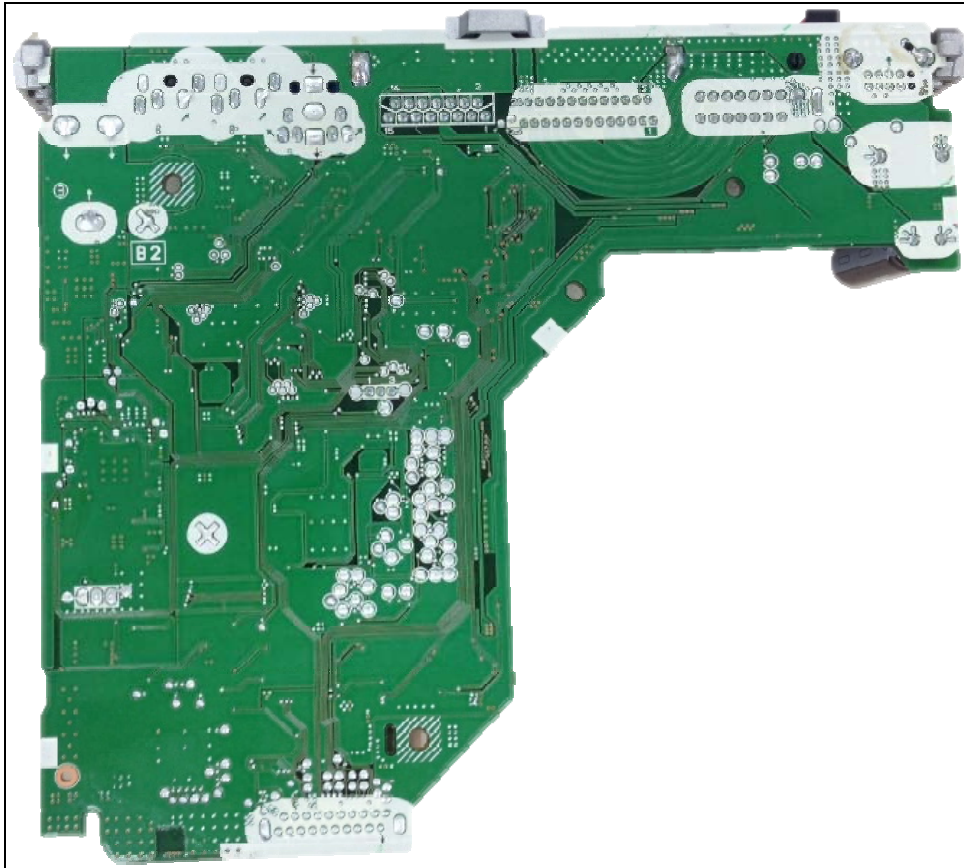
Bottom Side
